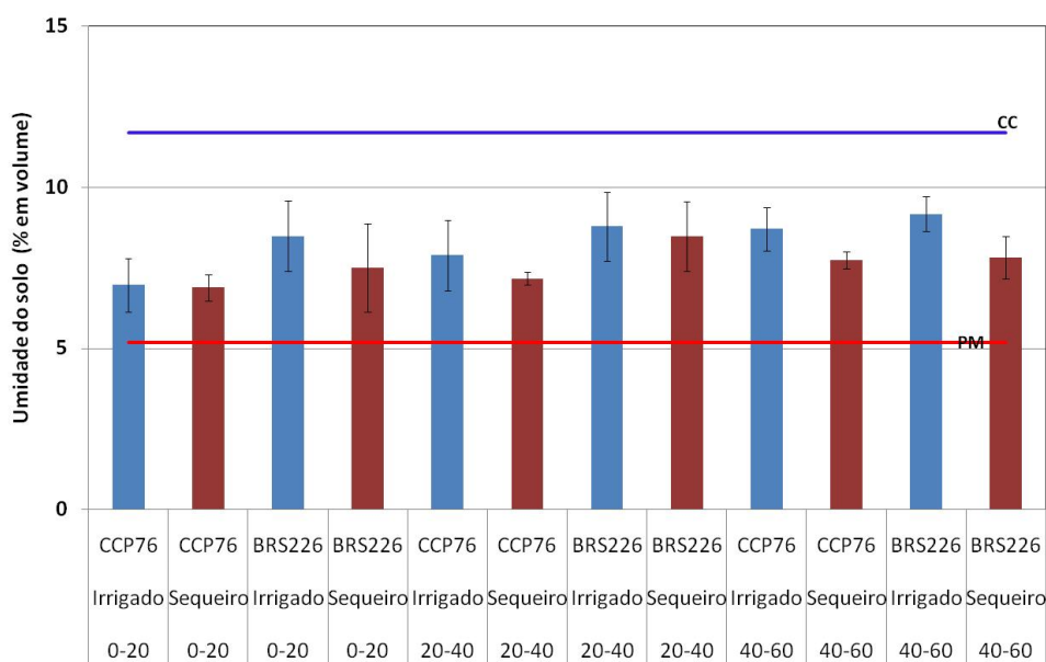
Figura 9 - Médias de umidade do solo (% em volume) nas camadas de 0-20, 20-40 e 40-60 cm na zona radicular de plantas de cajueiro dos clones CCP 76 e BRS 226, irrigadas e em sequeiro, na estação chuvosa (coleta realizada em 16/05/2019).
