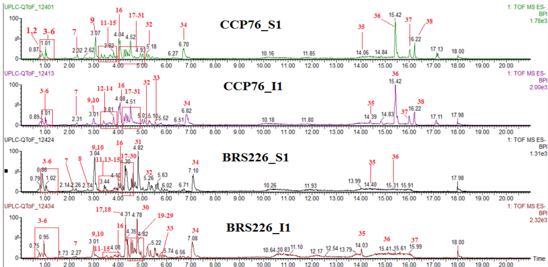
Figura 10 - Cromatogramas em modo BPI (Base Peak Intensity) referentes aos clones CCP76 e BRS 226 de cajueiro anão-precoce analisados, onde a sigla S1 significa sequeiro primeira coleta e I1 irrigado primeira coleta.
