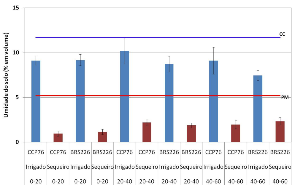
Figura 8 - Médias de umidade do solo (% em volume) nas camadas de 0-20, 20-40 e 40-60 cm na zona radicular de plantas de cajueiro dos clones CCP 76 e BRS 226, irrigadas e em sequeiro, no período de seca (coleta realizada em 30/11/2018). Onde a legenda PM significa: ponto de murcha e CC: capacidade de campo.
