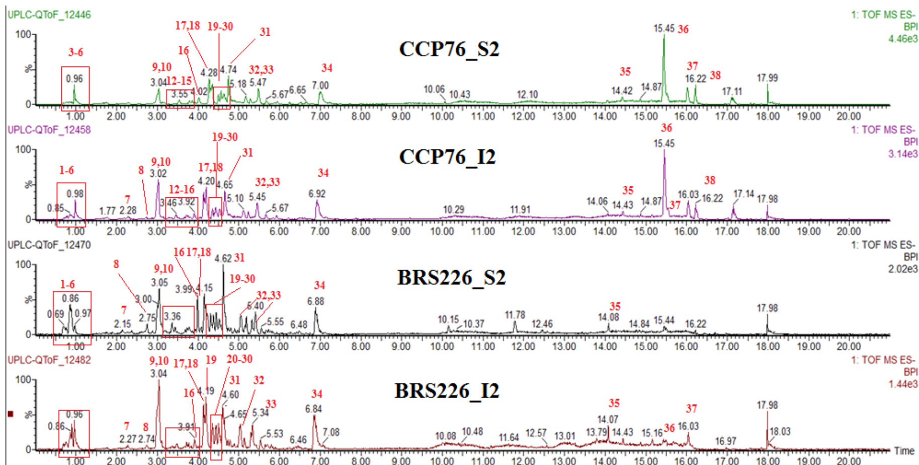
Figura 11 - Cromatogramas em modo BPI (Base Peak Intensity) referentes aos clones CCP76 e BRS 226 de cajueiro anão-precoce analisados, onde a sigla S2 significa sequeiro segunda coleta e I2 irrigado segunda coleta.
