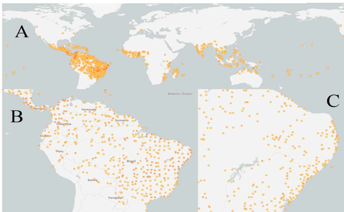
Figura 1 – Distribuição taxonômicas das ocorrências de Anacardium L catalogadas até 2019 (a) no mundo; (b) no Brasil e (c) no nordeste.
