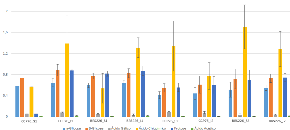
Figura 21 - Quantificações das principais variáveis latentes observadas na RMN ^1\text{H} , em mg/mL.
