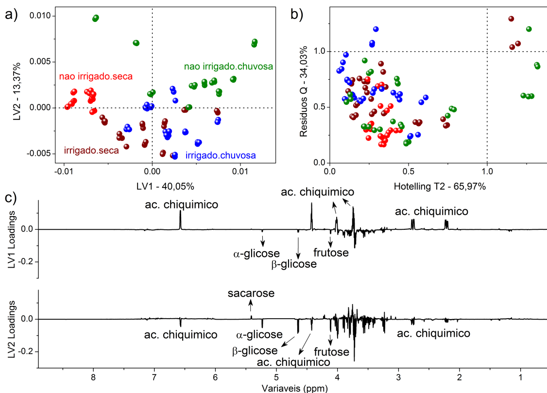
Figura 20 - a) Sistema de coordenadas de escores LV1 \times LV2 a partir da avaliação da sazonalidade e dos efeitos do estresse hídrico na variabilidade química das folhas de cajueiro dos genótipos BRS226; b) plotagem de influência da modelagem das amostras pelos resíduos T2 \times Q de Hotelling; c) respectivos loadings plotados em linhas com os compostos relevantes para a discriminação de amostras obtida por análise VIP.
