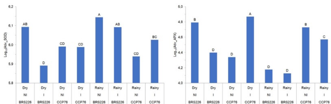
Figura 22 - Quantificações das enzimas APX e SOD, respectivamente. Valores contidos em \log_{10} para melhor visualização das diferenças. Teste de Tukey a 5 % de probabilidade.
