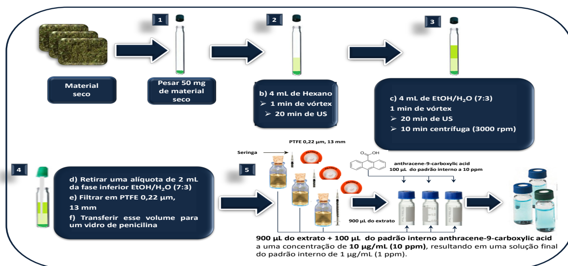
Figura 7 – Procedimento operacional padrão (POP) desenvolvido e utilizado na EMBRAPA para microextrações líquido-líquido para UPLC-QTOF-MS E .
