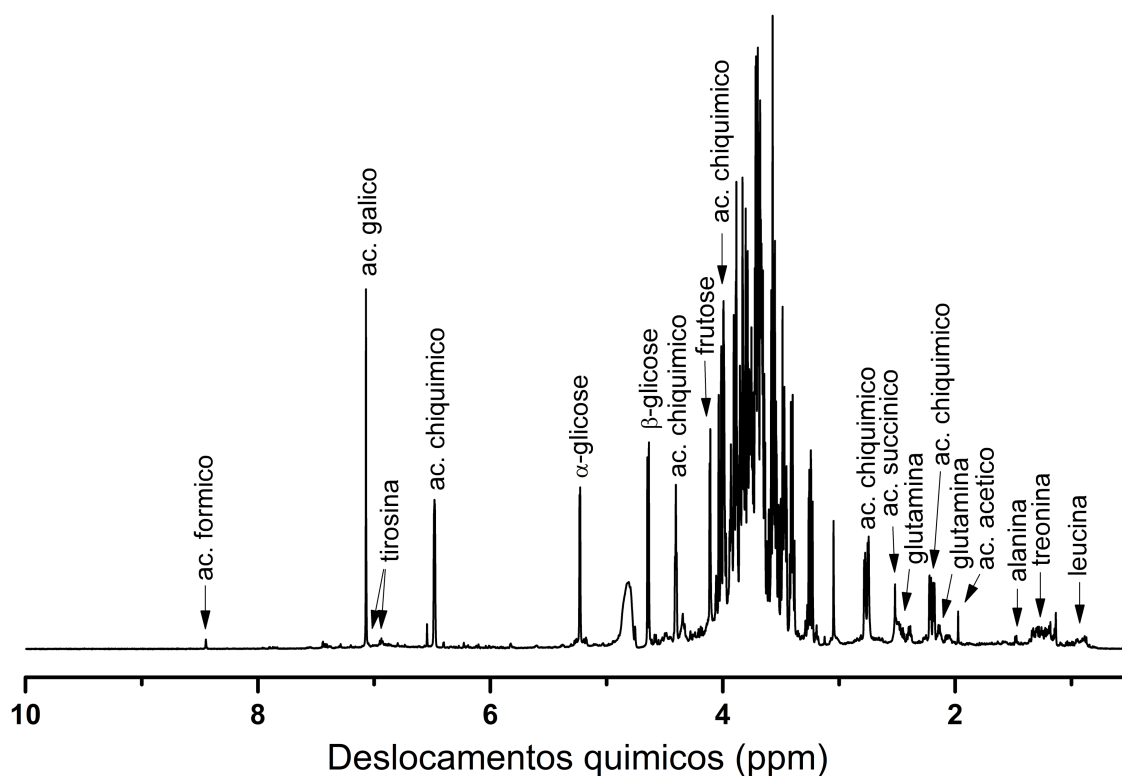
Figura 18 - Compostos identificados por RMN ^1\text{H} .
