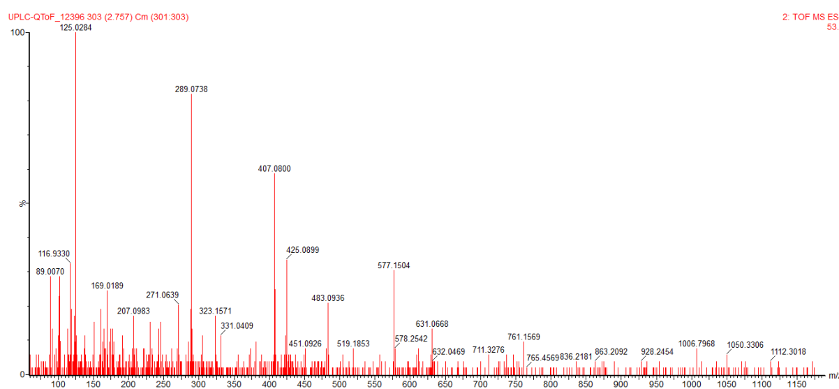
Figura 12 - Padrões de fragmentação da Procianidina tipo B.
