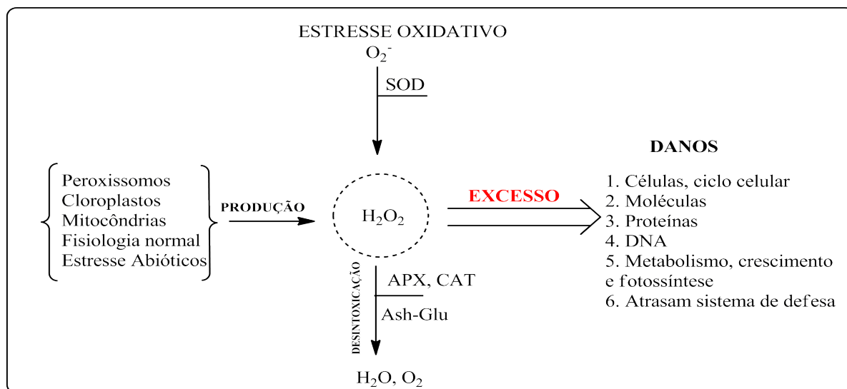
Figura 4 - Processo de desintoxicação do radical de oxigênio livre pelo sistema enzimático de defesa, suas fontes de origem e consequências do acúmulo de peróxido de hidrogênio nas células
