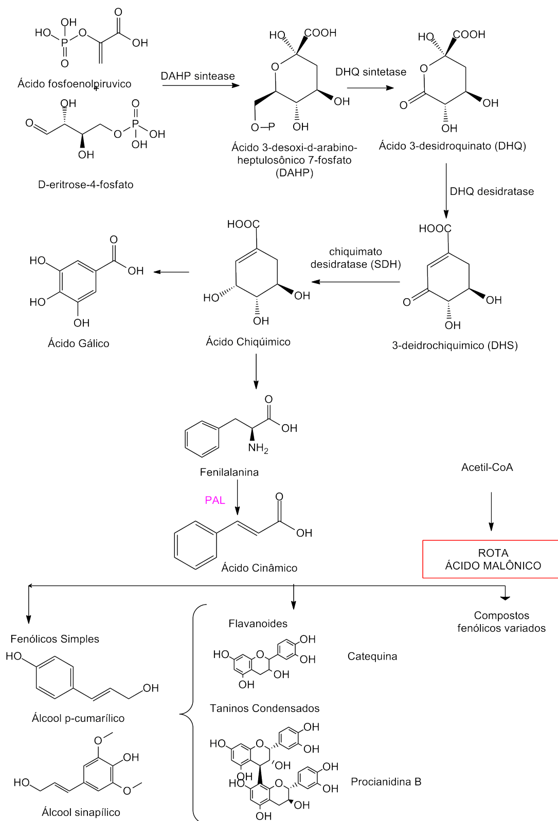
Figura 5 - Síntese do ácido chiquímico, seus principais produtos e derivados
