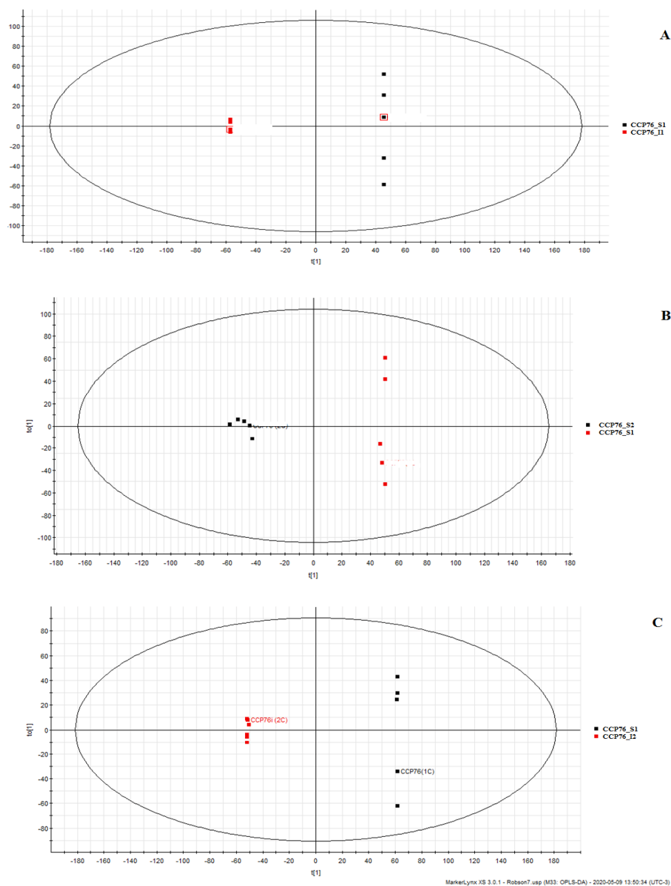
Figura 15 - Gráfico de scores OPLS-DA para os extratos de folhas da Anacardium Occidentale L. do clone CCP76: (A) CCP76_S1 x CCP76_I1; (B) CCP76_S1 X CCP76_S2; (C) CCP76_S1 x CCP76_I2
