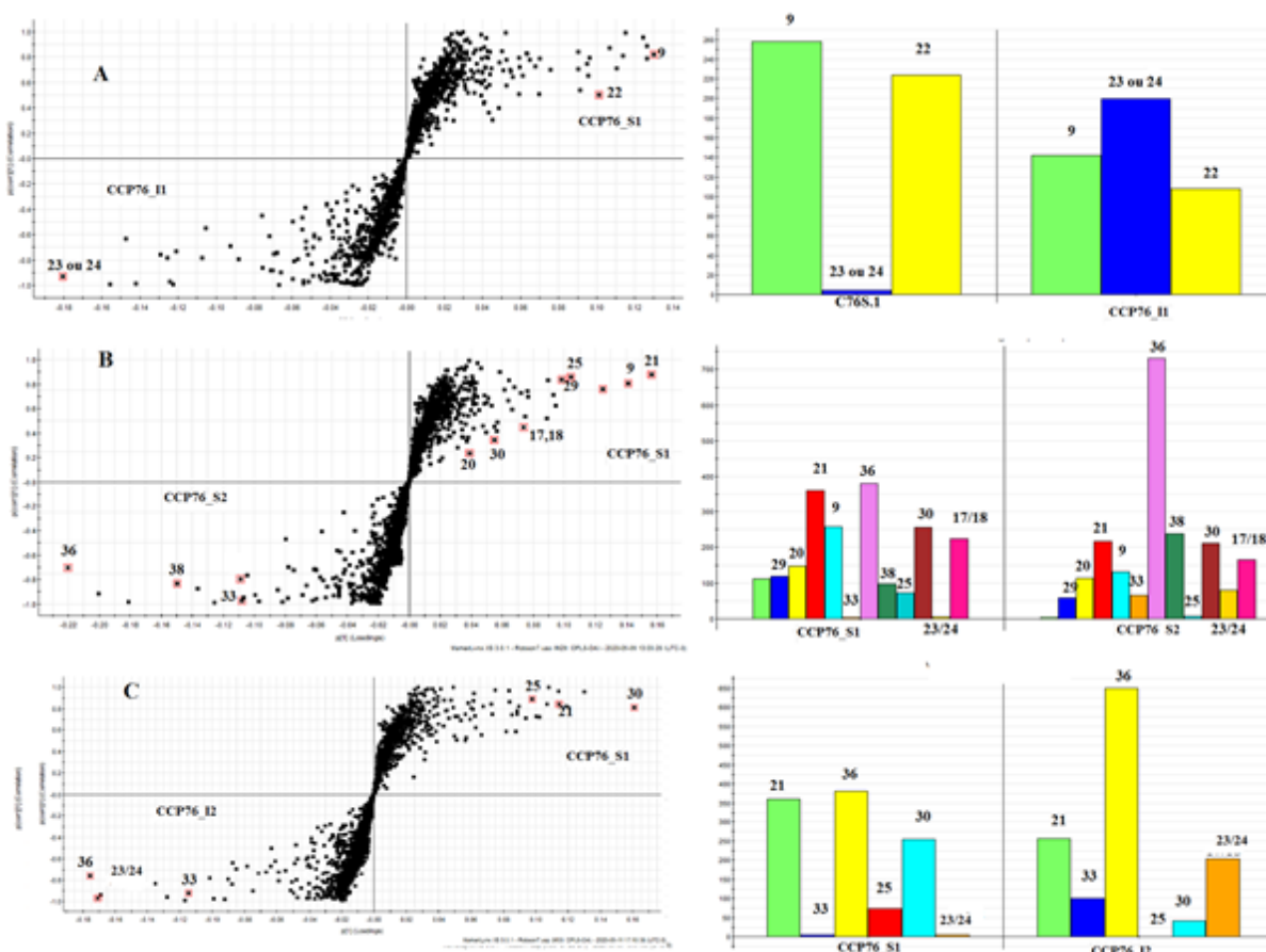
Figura 16 - Análise de S-Plot e gráficos de barras das duas variáveis de clone: (A) CCP76_S1 x CCP76_I1; (B) CCP76_S1 X CCP76_S2; (C) CCP76_S1 x CCP76_I2.
