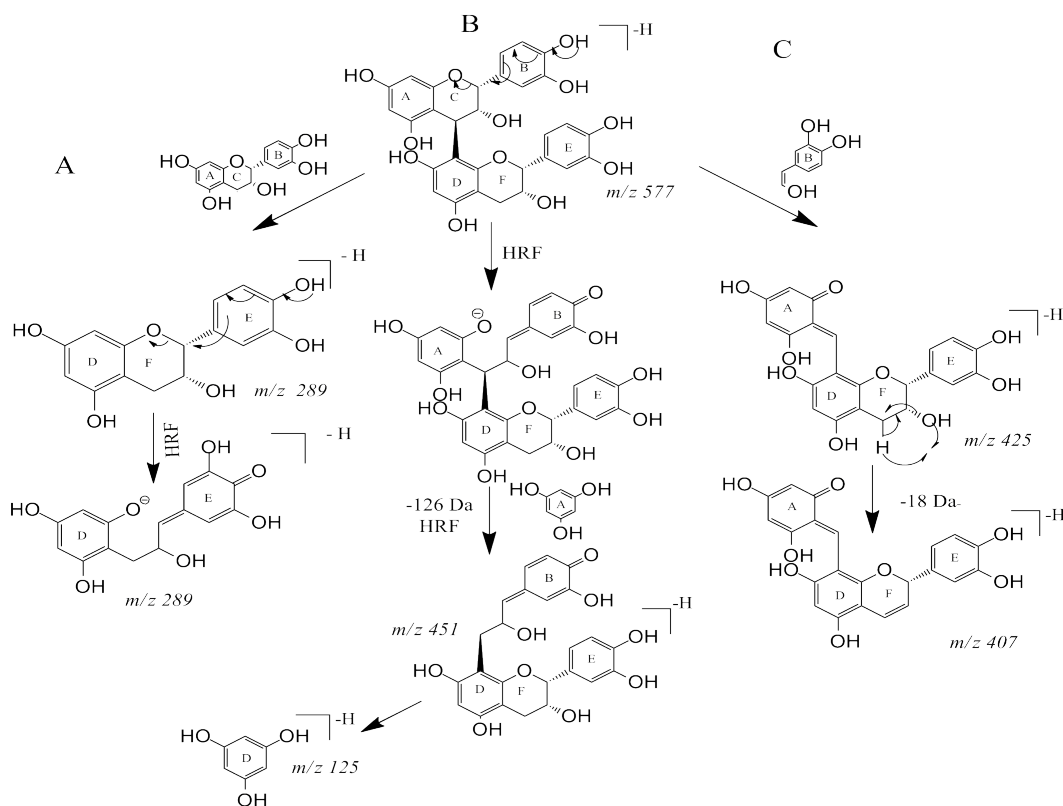
Figura 13 - Principais fragmentações de procianidina do tipo B em modo negativo [M-H]^- : (A) Fragmentação quinona metideo, (B) fissão heterocíclica do anel e (C) Retro Diels Alder.
