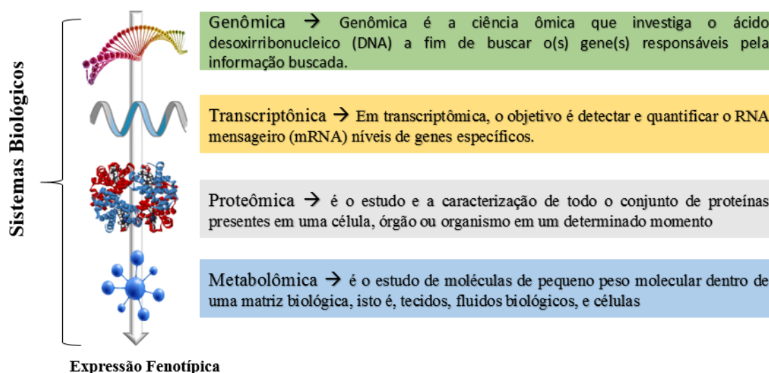
Figura 2 - Representação da cascata ômica
