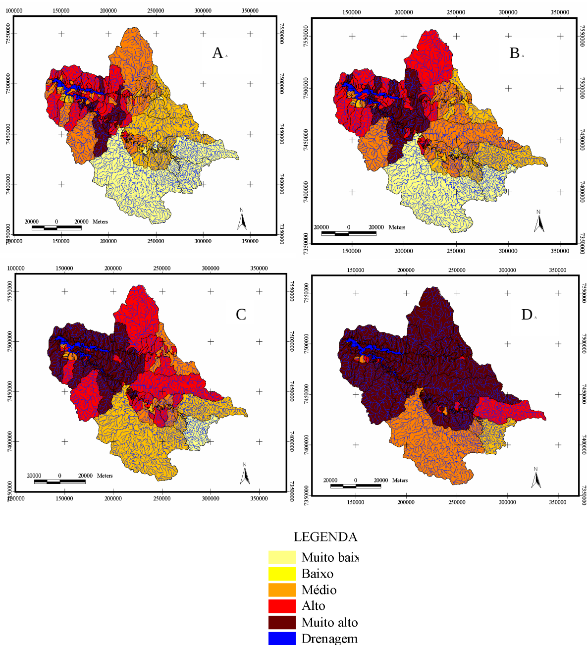
Figura 3: Mapas representando os Cenários obtidos a partir da modelagem sendo A – Cenário 1 (Peso 3), B Cenário 2 (Peso 4), C - Cenário 3 (Peso 5), D – Cenário 4 (Peso 7).
