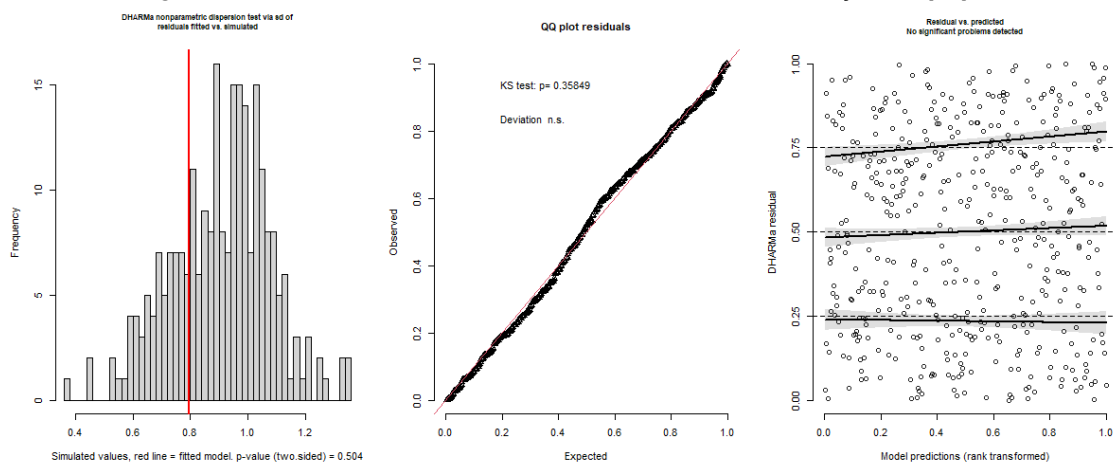
Figura S20. Análise visual dos resíduos do modelo de extração de piquiá .
