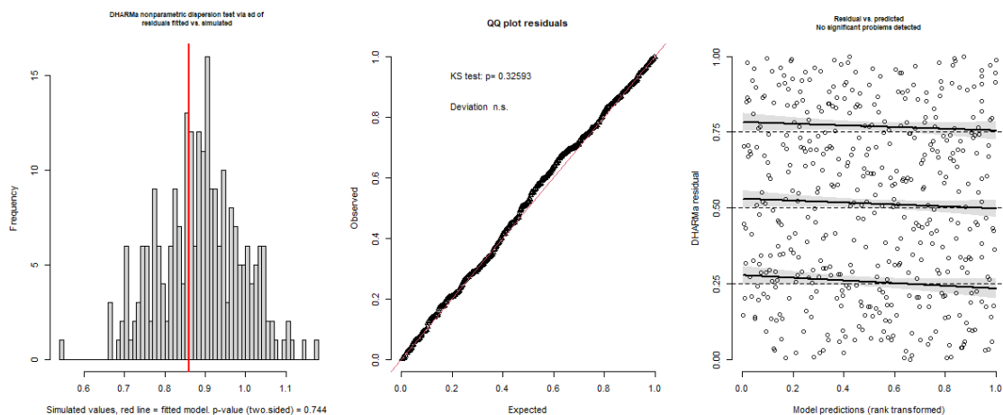
Figura S16. Análise visual dos resíduos do modelo de extração de castanha .
