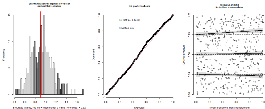
Figura S15. Análise visual dos resíduos do modelo de extração de andiroba .
