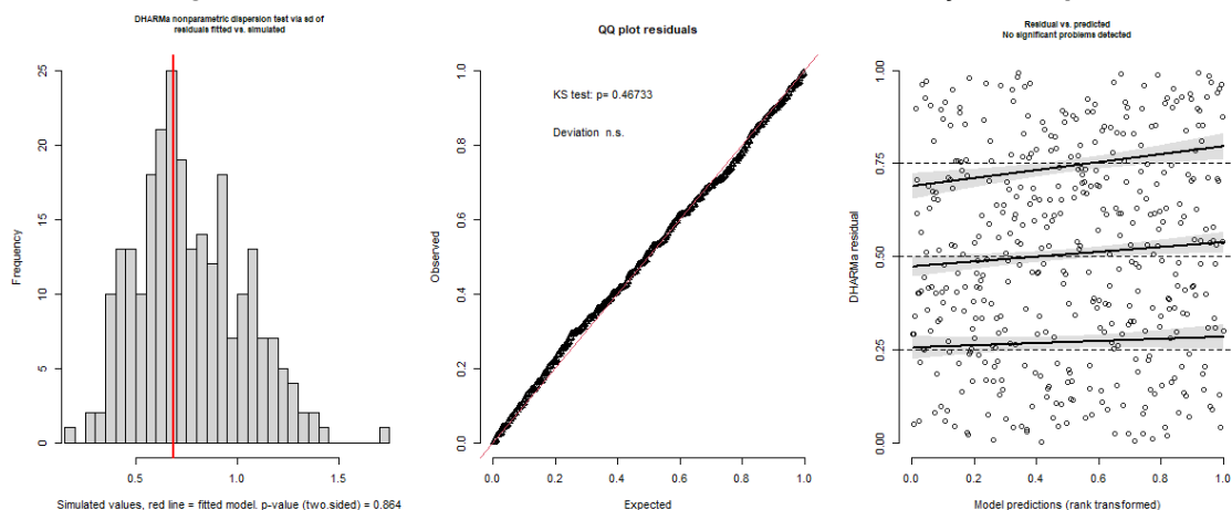
Figura S17. Análise visual dos resíduos do modelo de extração de cipó .
