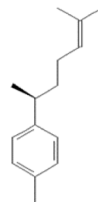
(+)\text{-}\alpha\text{-curcumene}
