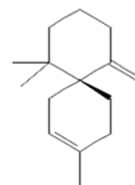
\beta\text{-chamigrene}
