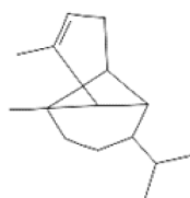
\alpha\text{-copaene}
