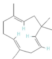
\alpha\text{-humulene}
