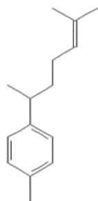
\alpha\text{-curcumene}
