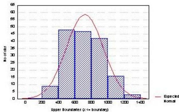
Figura 2 – Histograma dos valores do percentil 75 da precipitação anual
