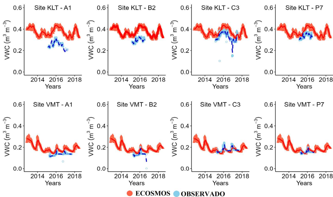
Figura 1: Teor Volumétrico de Água do Solo (VWC, m^3 m^{-3} ) para a profundidade de 0 – 3 metros para os sítios de Bocaiuva – MG (VMT) e Telêmaco Borba – PR (KLT) quando cultivados com E. urophylla (A1), E. urophylla x E. grandis (B2), Eucalyptus grandis x camaldulensis (C3) e E. urophylla x E. brassiana (P7). Círculos azuis correspondem aos valores observados e círculos vermelhos aos simulados.
