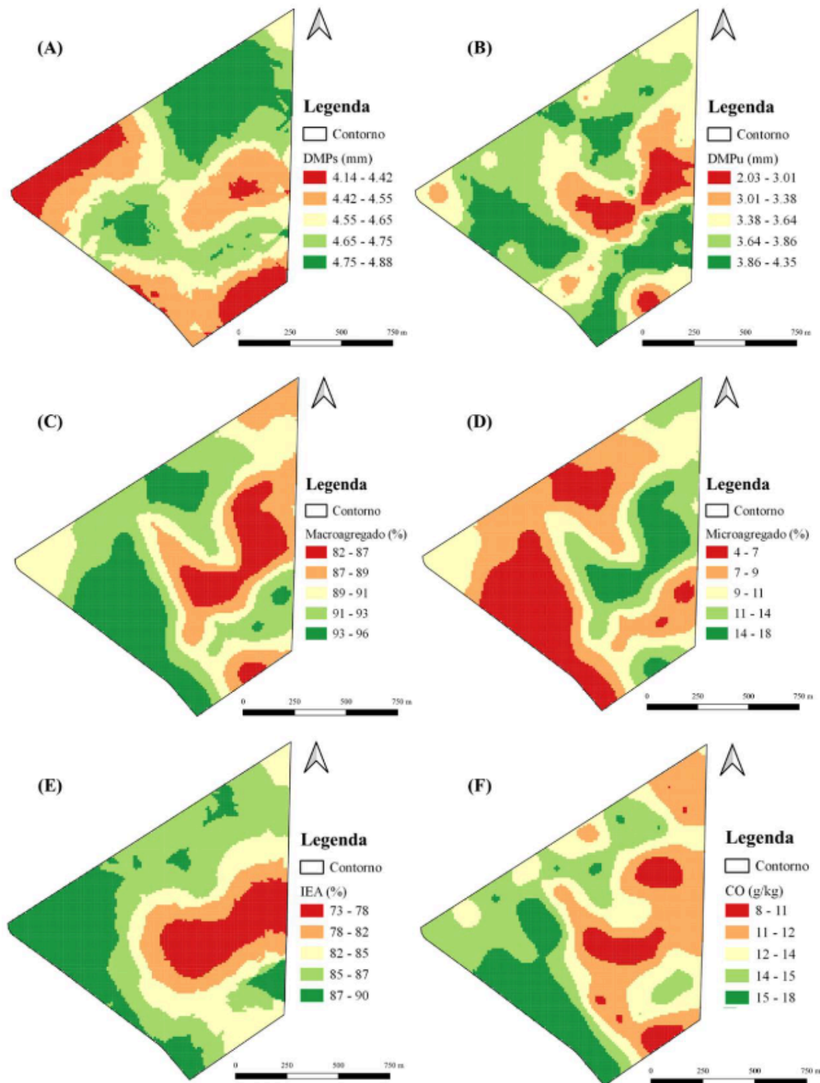
Figura 6. Mapas de variabilidade espacial dos atributos diâmetro médio ponderado seco (A), diâmetro médio ponderado úmido (B), macroagregados (C), microagregados (D), IEA - índice de estabilidade dos agregados (E) e carbono orgânico (F).
