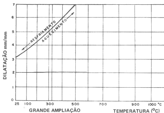
CURVA HIDRODILATOMETRIA DA CÁPSULA
