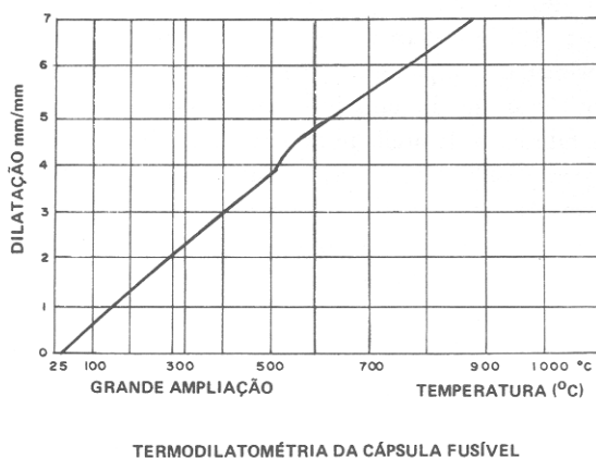
FIG. 1. Curva termodilatométrica do material usado para confecção das cápsulas porosas.
