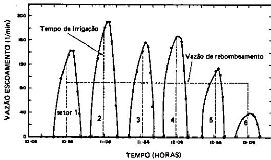
FIG. 6. Hidrógrafas da vazão de escoamento por setor no sistema de recirculação de água de irrigação com bombeamento contínuo para R igual a 0,50.
