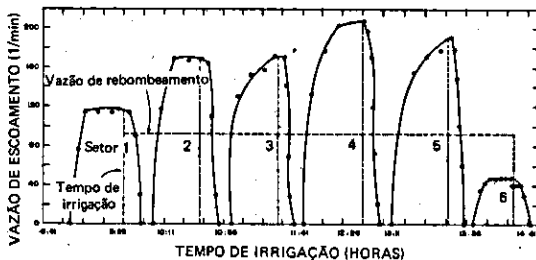
FIG. 8. Hidrógrafas da vazão de escoamento por setor no sistema de recirculação de água de irrigação com bombeamento contínuo para R igual a 2.
