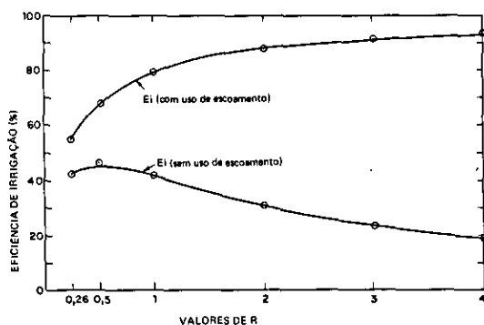
FIG. 10. Eficiência de irrigação com e sem reuso da água de escoada versus valores de R .
