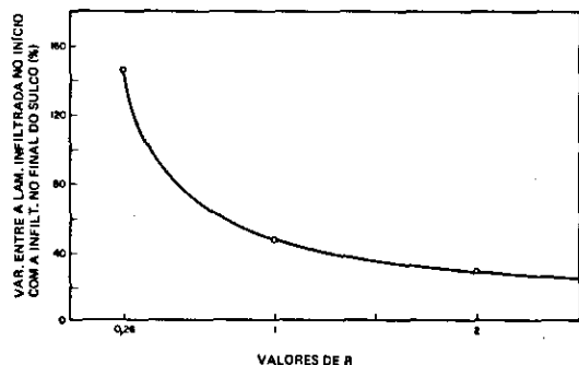
FIG. 4. Variação da lâmina infiltrada no início com a infiltrada no final do sulco versus valores de R .
