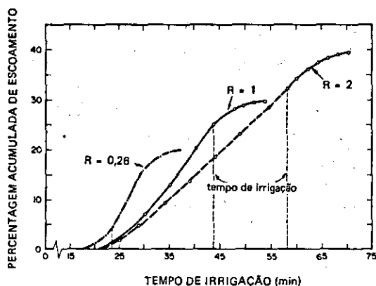
FIG. 5. Percentagem média acumulada de escoamento em relação ao tempo de irrigação para o sistema de irrigação com sifão, para R iguais a 0,26; 1 e 2.
