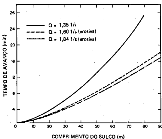
FIG. 2. Curvas de avanço para as vazões de 1,35; 1,60 e 1,84 l/s para uma declividade de sulco de 0,27% para um oxissol unidade 37BB.
