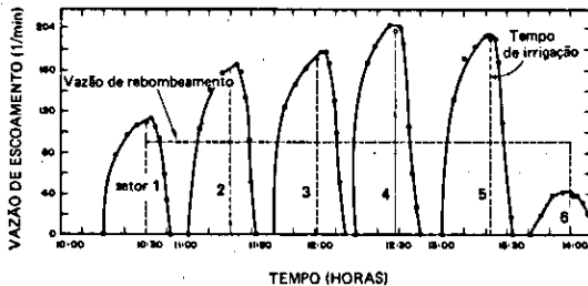
FIG. 7. Hidrógrafas da vazão de escoamento por setor no sistema de recirculação de água de irrigação com bombeamento contínuo para R igual a 1.
