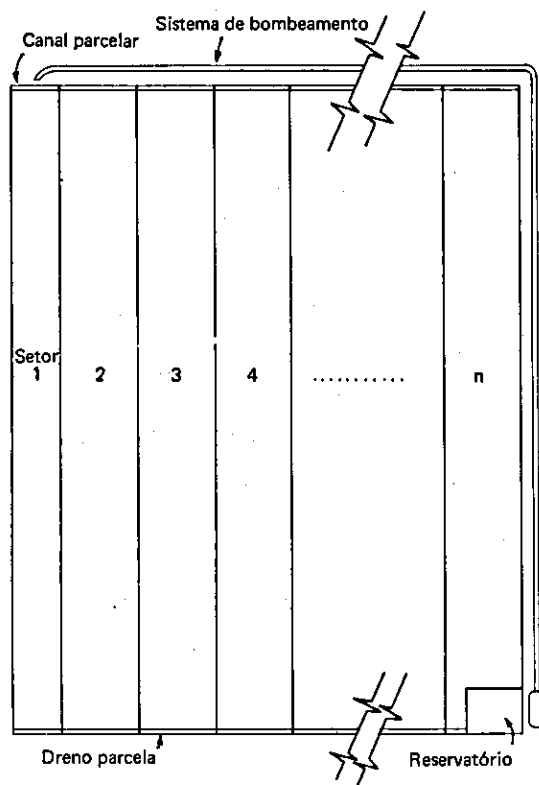
FIG. 1. Esquema de um sistema de irrigação típico com utilização da água escoada.
