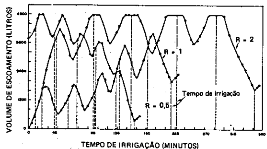
FIG. 9. Hidrógrafas do volume de escoamento disponível no reservatório no sistema de irrigação com utilização da água escoada com bombeamento contínuo para valores de R igual a 0,5; 1 e 2.
