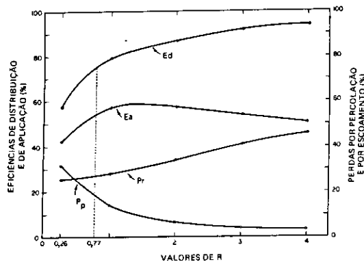
FIG. 3. Curvas de perdas de água por percolação (Pp) e por escoamento superficial (Pe) e eficiências de distribuição (Ed) e de aplicação (Ea) em função de R.
