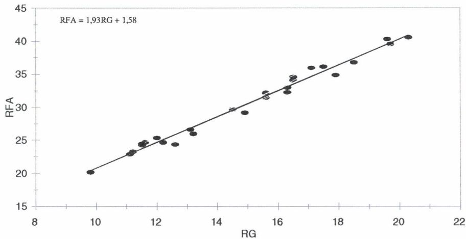
Fig.1. Relação entre a radiação fotossinteticamente ativa (RFA) e radiação solar global (RG) em Petrolina-PE, no período de 1 de junho a 31 de julho de 1994 ( r^2 = 0,98 ).
