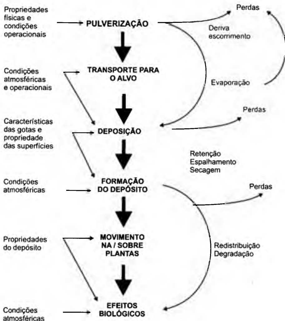
Fig. 1. Dinâmica do processo de pulverização foliar.
