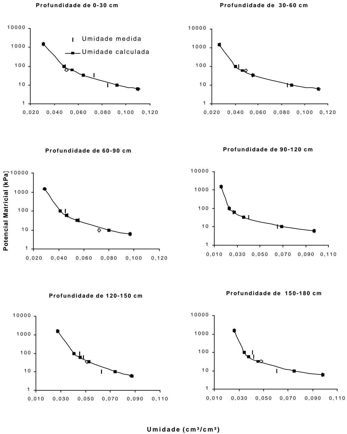
FIGURA 1 - Curvas características de água no solo da fazenda São João, devidamente ajustadas pelo modelo Van Genuchten, referente à Planta 1.
