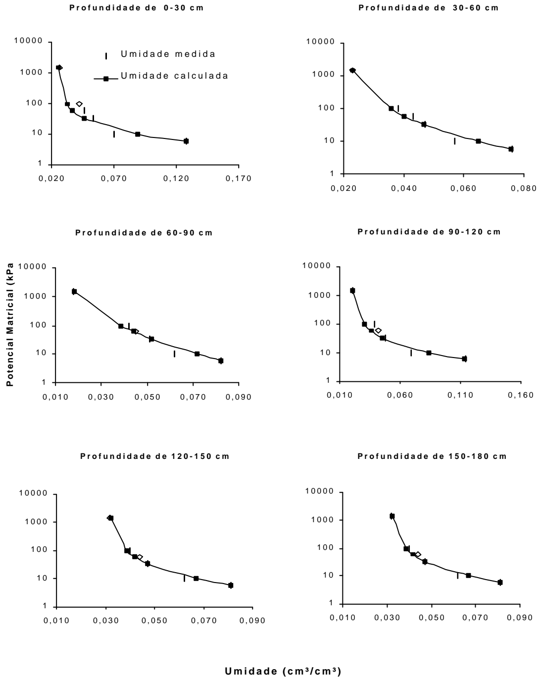
FIGURA 2- Curvas características de água no solo da fazenda São João, devidamente ajustadas pelo modelo Van Genuchten, referente à Planta 2.
