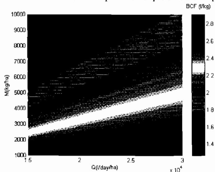
FIGURA 3. Influencia de M y Q de plantas de mangos en el cálculo del BCF de paclobutrazol simulado por el modelo FTM-p.
