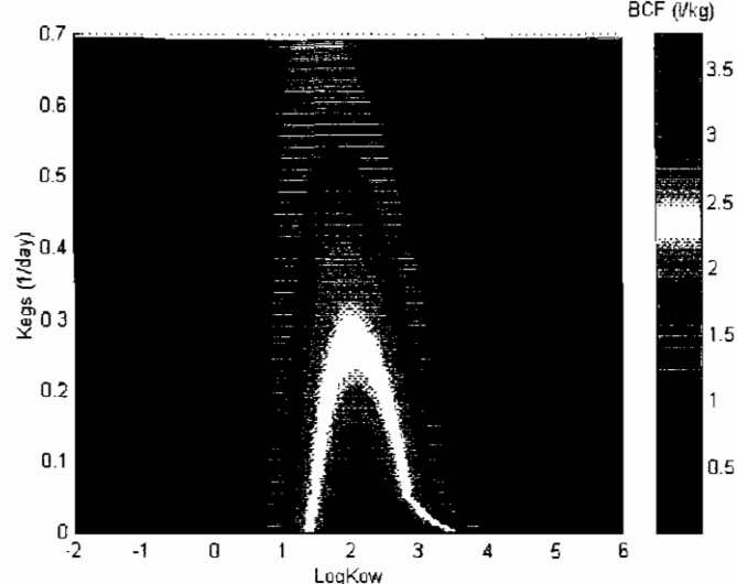
FIGURA 4. Influencia de \log K_{OW} y k_{EGS} en el claculo del BCF de paclobutrazol simulado por el modelo FTM-p.
