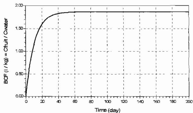
FIGURA 2. Simulación con el modelo FTM-p del BCF de paclobutrazol en plantas de mangos.
