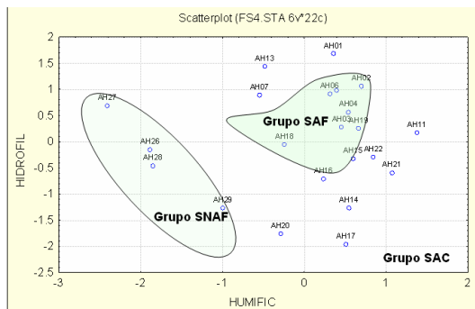
Figura 02. Agrupamento dos ácidos húmicos estudados em função dos fatores humificação e hidrofiliçidade, após a remoção do efeito das cinzas.
