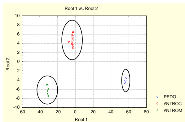
Figura 04. Agrupamento dos ácidos húmicos em função das duas primeiras variáveis discriminantes. Root 1 e 2: variáveis discriminantes 1 e 2, respectivamente.
