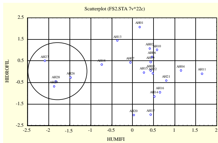
Figura 01. Agrupamento dos ácidos húmicos estudados em função dos fatores humificação e hidrofilicidade
