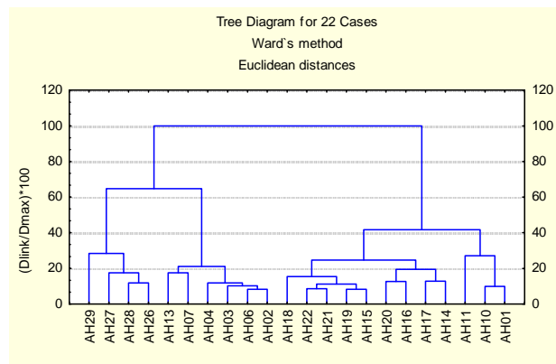
Figura 03. Grupamento hierárquico dos ácidos húmicos estudados.
