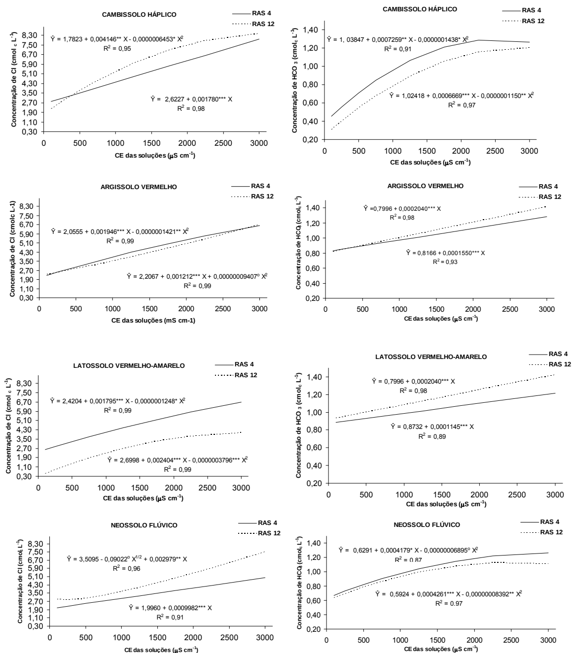
Figura 4. Equações de regressão das variáveis dos teores de \text{Cl}^- e \text{HCO}_3^- do lixiviado coletado aos 30 dias do experimento nos quatro solos estudados em função da CE das soluções de percolação.
