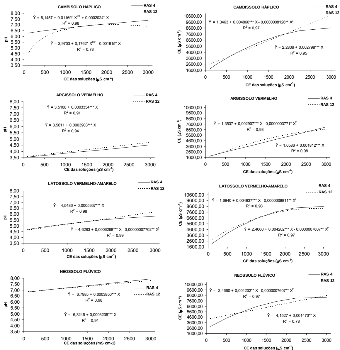
Figura 1. Equações de regressão das variáveis de pH, condutividade elétrica (CE), do lixiviado coletado aos 30 dias do experimento nos quatro solos estudados em função da CE das soluções de percolação.
