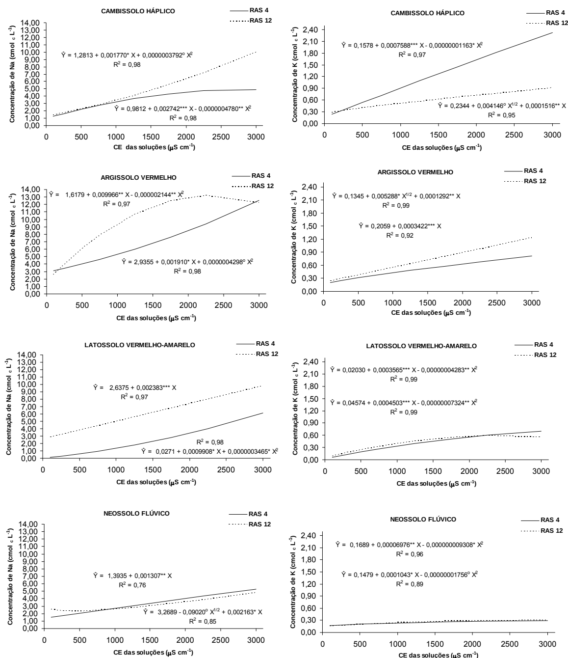
Figura 3. Equações de regressão das variáveis dos teores de Na + e K + do lixiviado coletado aos 30 dias do experimento nos quatro solos estudados em função da CE das soluções de percolação.
