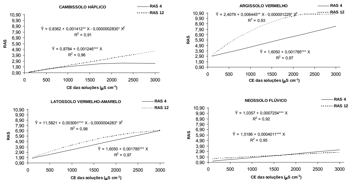
Figura 5. Equações de regressão da relação de adsorção de (RAS) do lixiviado coletado aos 30 dias do experimento nos quatro solos estudados em função da CE das soluções de percolação.
