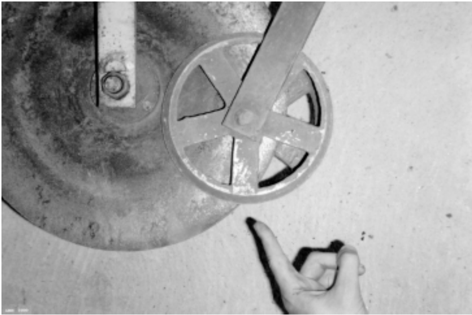
Figura 1. Detalhe do encaixe do disco de corte na roda limitadora de profundidade.
