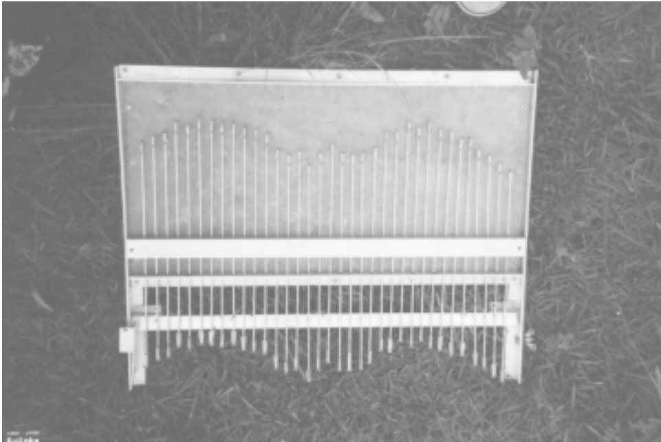
Figura 1. Vista geral do perfilógrafo desenvolvido para avaliar a mobilização do solo.
