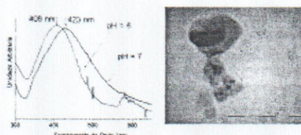
Figura 1. Os picos nos espectros de UV-visível indicam a formação de suspensões coloidais de prata e o deslocamento para o azul em função do menor pH indica que foram obtidas partículas de menor tamanho (20 nm para pH = 6 e 60 nm para pH = 7). A imagem de microscopia eletrônica de transmissão mostra um aglomerado de nanopartículas de prata sintetizadas com pH inicial de 7.
