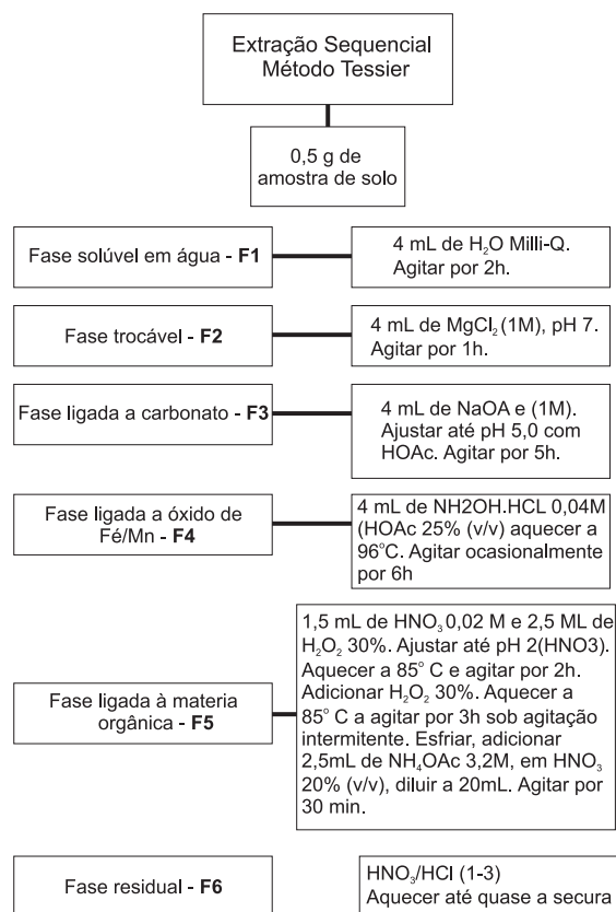
Figura 2. Fluxograma com as etapas e os reagentes utilizados na extração sequencial segundo Tessier
