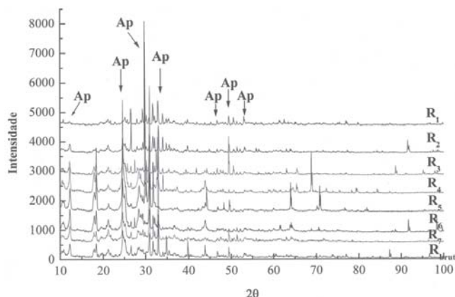
Figura 1. Difratogramas de raios-X das amostras peneiradas (R1 <0,074; R2 0,074 – 0,125; R3 0,125 – 0,177; R4 0,177 – 0,210; R5 0,210 – 0,250; R6 > 0,250; R7 <0,210 e R8 rocha bruta)
