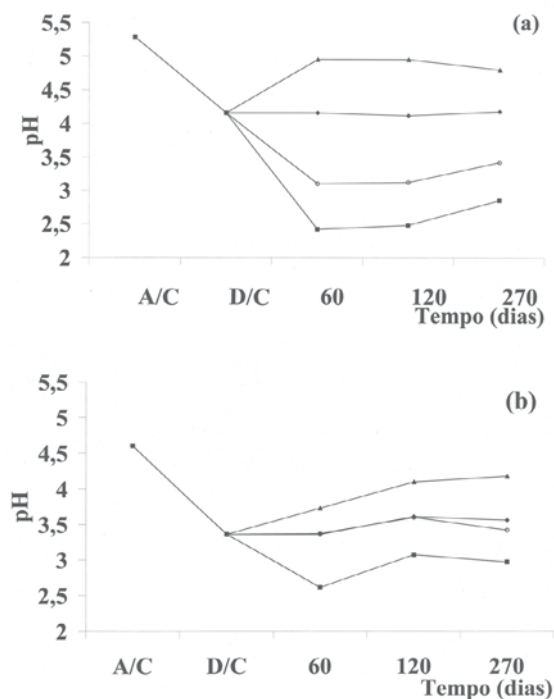
Figura 3. Valores do pH antes da contaminação (A/C), depois da contaminação com chumbo (D/C), 60, 120 e 270 dias após os tratamentos: T0 (◆); T1 (■); T2 (▲) e T3 (○). LA (a) e LV (b)
