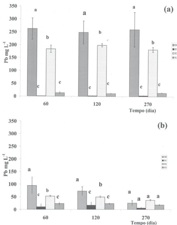
Figura 4. Concentrações de Pb após extração por TCLP em amostras de solos LA (a) e LV (b) coletadas em 60, 120 e 270 dias após os tratamentos. Letras minúsculas diferentes representam diferença significativa ( P < 0,05 ) pelo teste de Tukey
