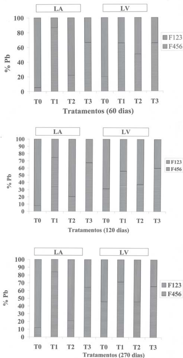
Figura 6. Extração sequencial após 60 (a), 120 (b) e 270 (c) dias da realização dos tratamentos (T0 - solo sem tratamento; T1 - H 3 PO 4 ; T2 - rocha; T3 - H 3 PO 4 e rocha)
