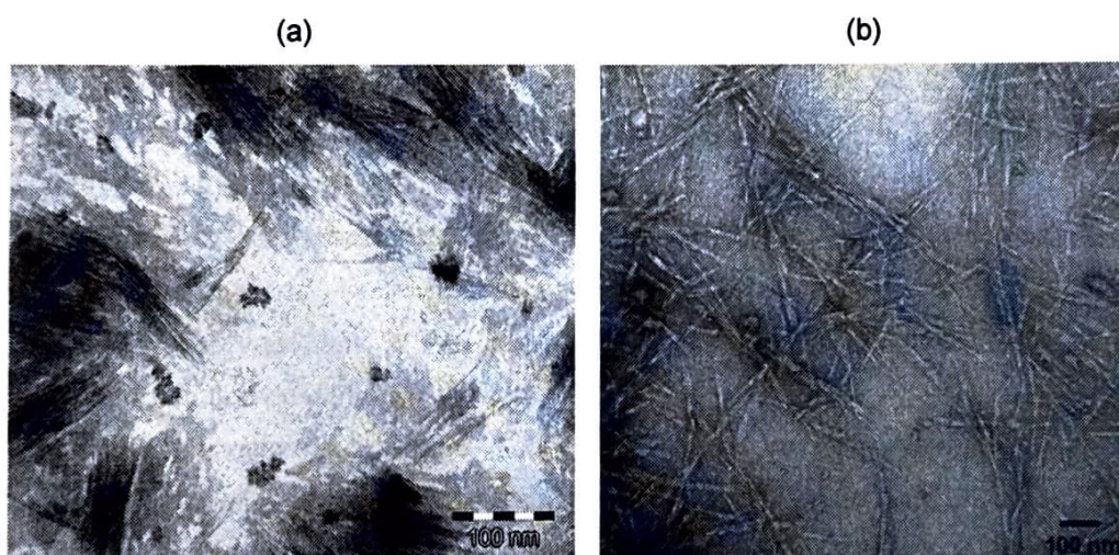
Fig. 3a,b - Whiskers de celulose extraídos de fibras de coco imaturo previamente branqueadas (a: tratamento T2 e hidrólise ácida de 120 min, b: tratamento T1) e hidrólise ácida de 90 min.
