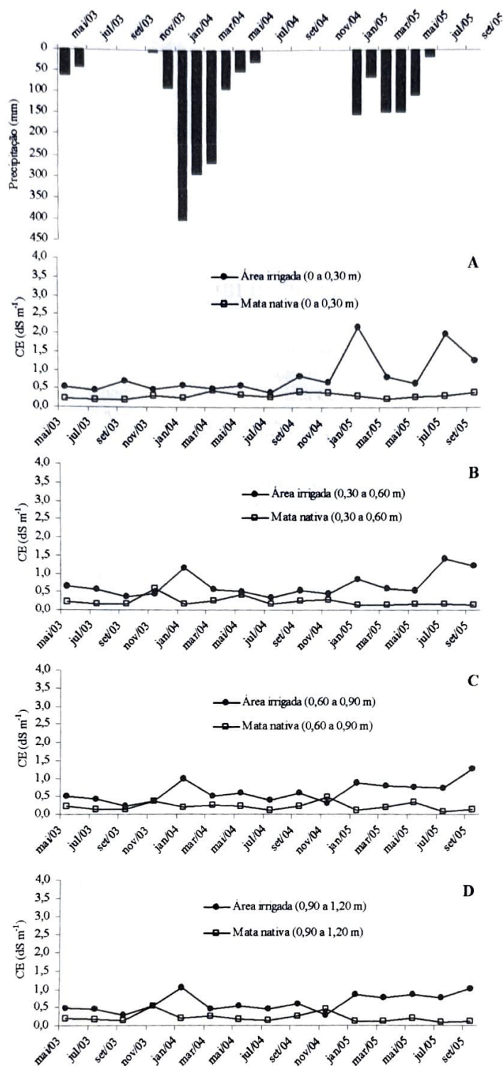
Figura 1. Variação espaço-temporal da condutividade elétrica no solo do Distrito de Irrigação do Perímetro Araras Norte, Ceará.
