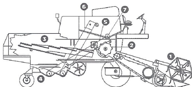
FIGURA 1 | CONSTITUIÇÃO DE UMA COLHEDORA AUTOMOTRIZ
