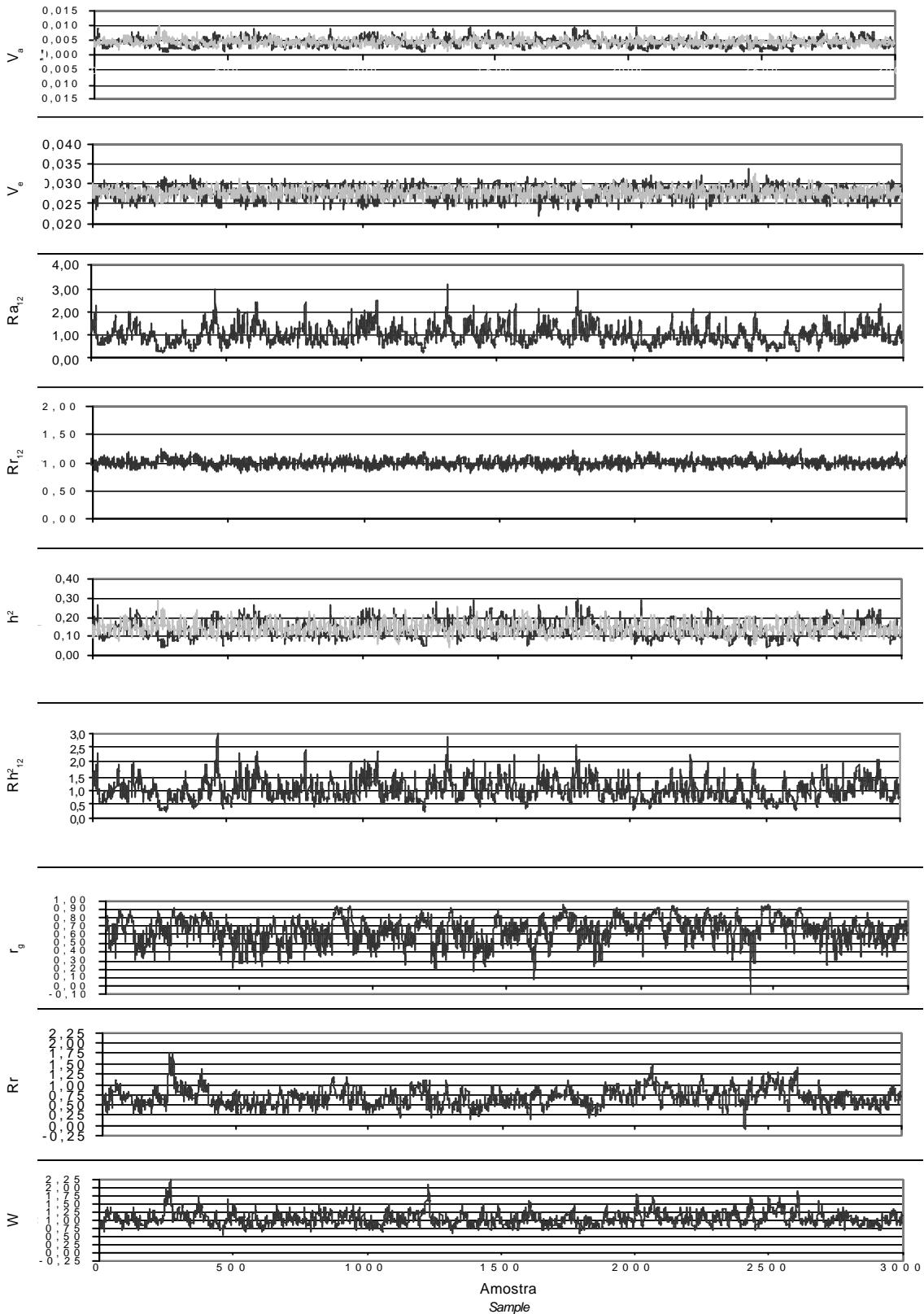
Figura 2 - Histórico da amostragem das variâncias aditiva direta ( V_a ) e residual ( V_e ), razões das variâncias aditivas diretas ( R_{a_{12}} ) e residuais ( R_{r_{12}} ), herdabilidade ( h^2 ), razão de herdabilidades ( Rh^2_{12} ), correlação genética ( r_g ), resposta relativa da seleção indireta ( Rr = h_1 \cdot h_2 \cdot r_g / h^2_1 ) e eficiência relativa da seleção sem interação ( W = h_2/h_1 ) para o ganho diário da desmama aos 12 meses de idade. Para V_a , V_e e h^2 , a cor preta refere-se à época 1 e a cinza, à época 2.
