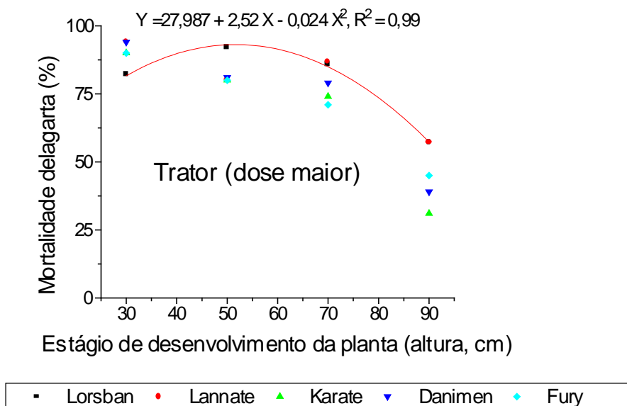
Figura 2. Curva ajustada de mortalidade de diferentes inseticidas (dose 50% acima da recomendada), aplicados com trator em plantas de milho de diferentes estádios de desenvolvimento. Sete Lagoas, MG.
