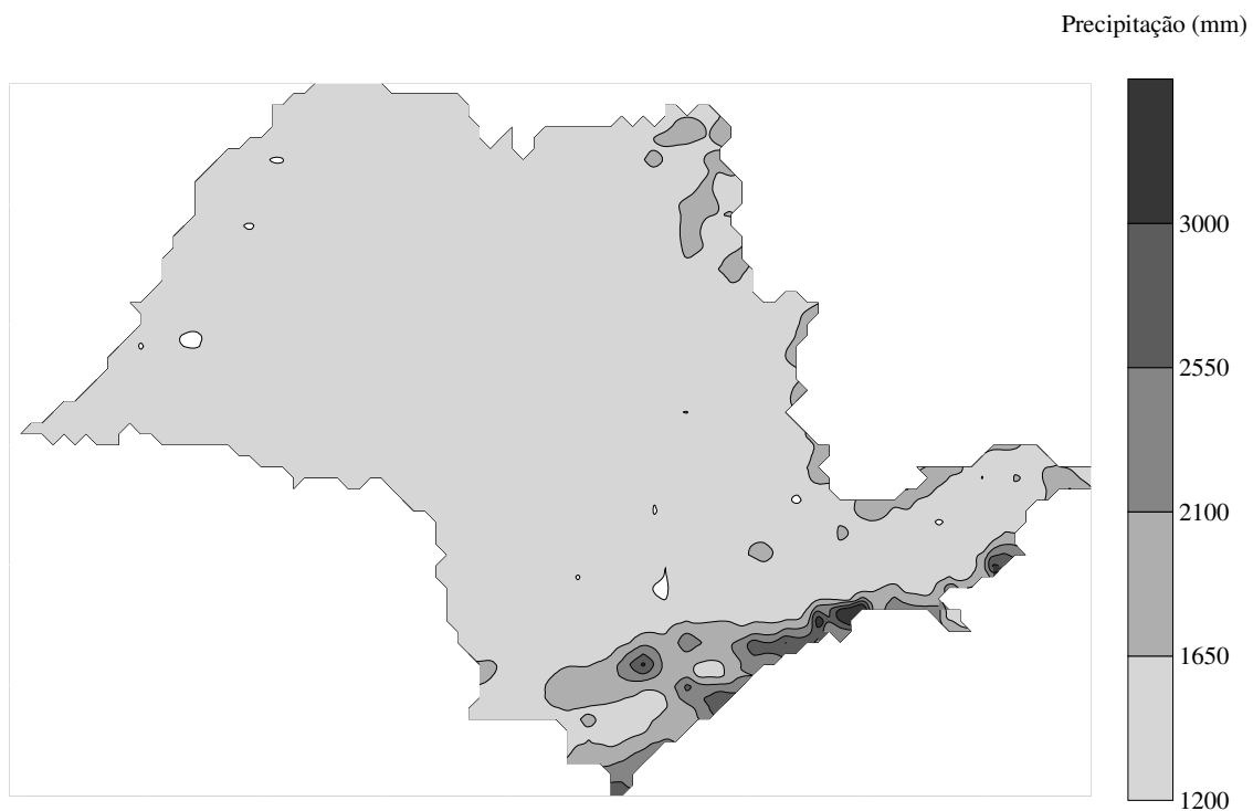
FIGURA 5. Distribuição espacial para precipitação pluviométrica média anual no Estado de São Paulo obtida por meio da curvatura mínima.
