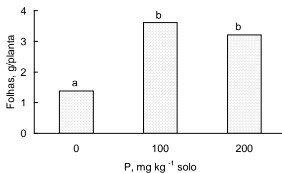
Figura 27. Efeito da adição de P no solo sobre a produção de matéria seca de folhas de mudas de Sclerolobium paniculatum em Latossolo Vermelho Escuro aos 230 dias após a semeadura. Médias seguidas pela mesma letra não diferem significativamente pelo teste de Tukey a 5%.
