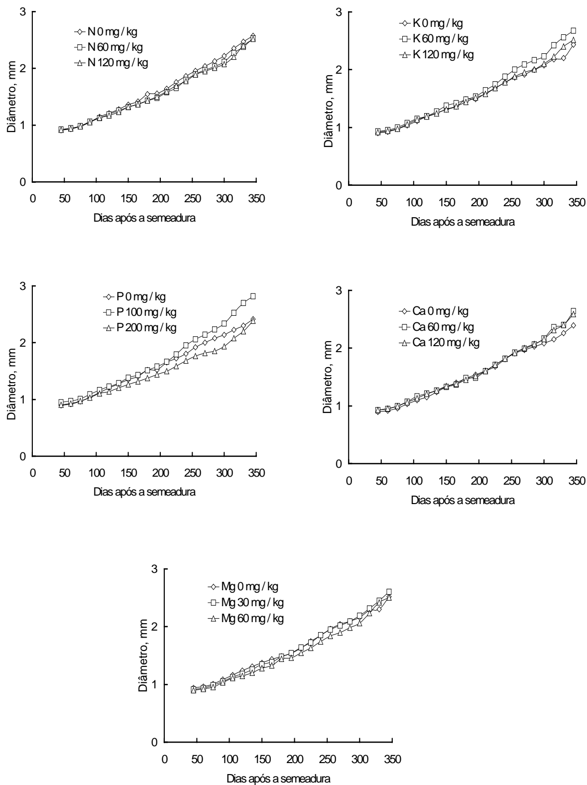
Figura 4. Efeito da adição de nutrientes no solo sobre o diâmetro do colo de mudas de Eugenia dysenterica em Latossolo Vermelho Escuro até 345 dias após a semeadura.
