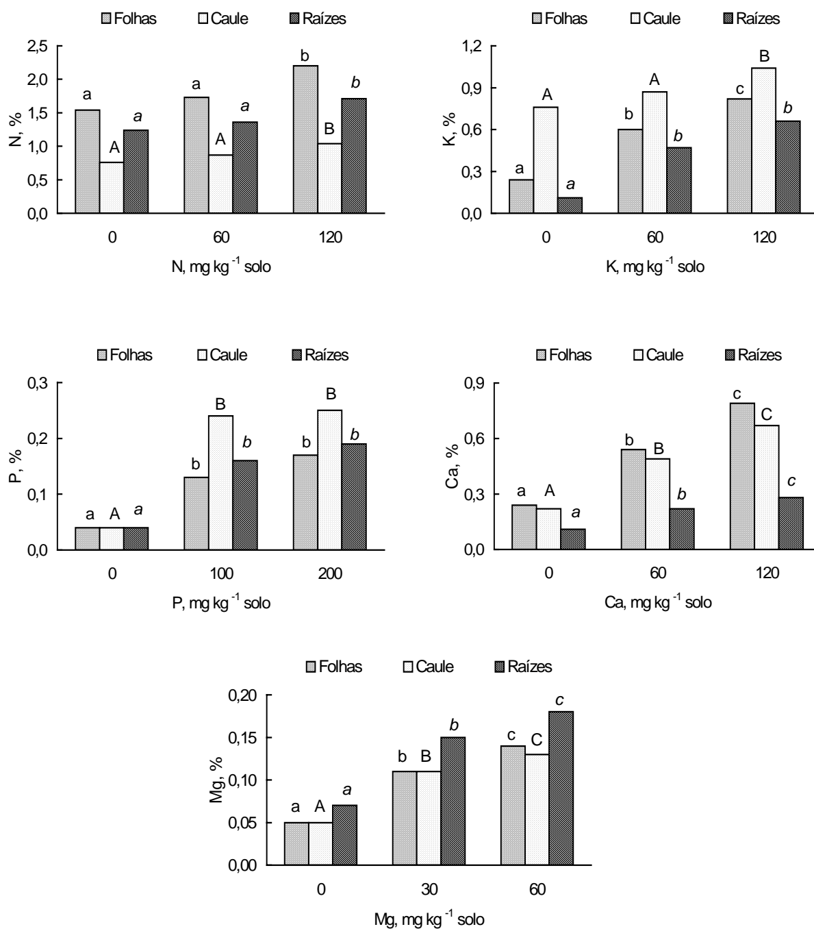
Figura 32. Efeito da adição de N, P, K, Ca e Mg no solo sobre a concentração do próprio elemento nas folhas, caule e raízes de mudas de Sclerobolium paniculatum em Latossolo Vermelho Escuro aos 230 dias após a semeadura. Médias seguidas pela mesma letra para o mesmo componente não diferem significativamente pelo teste de Tukey a 5%.
