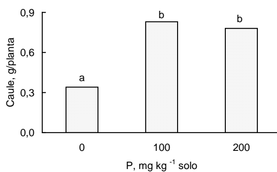
Figura 28. Efeito da adição de P no solo sobre a produção de matéria seca do caule de mudas de Sclerolobium paniculatum em Latossolo Vermelho Escuro aos 230 dias após a semeadura. Médias seguidas pela mesma letra não diferem significativamente pelo teste de Tukey a 5%.
