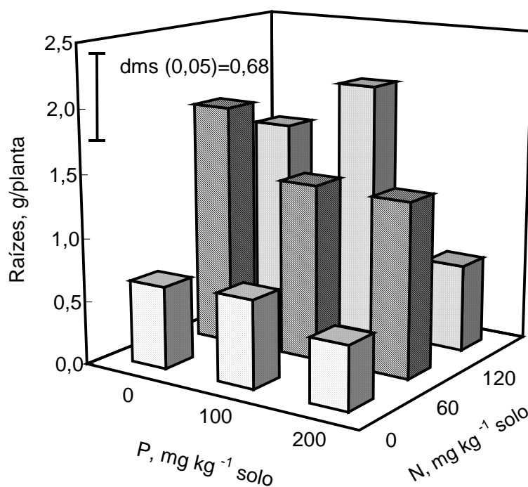
Figura 30. Efeito da adição de N e P no solo sobre a produção de matéria seca das raízes de mudas de Sclerobium paniculatum em Latossolo Vermelho Escuro aos 230 dias após a semeadura (dms = diferença mínima significativa ao nível de 5%).
