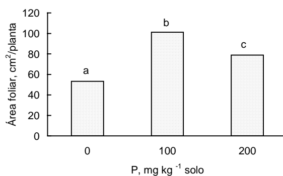
Figura 9. Efeito da adição de P no solo sobre a área foliar de mudas de Eugenia dysenterica em Latossolo Vermelho Escuro 345 dias após a semeadura. Médias seguidas pela mesma letra não diferem significativamente pelo teste de Tukey a 5%.
