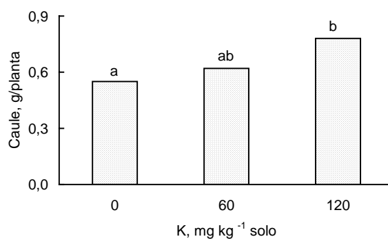
Figura 29. Efeito da adição de K no solo sobre a produção de matéria seca do caule de mudas de Sclerolobium paniculatum em Latossolo Vermelho Escuro aos 230 dias após a semeadura. Médias seguidas pela mesma letra não diferem significativamente pelo teste de Tukey a 5%.
