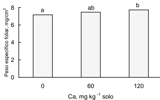
Figura 56. Efeito da adição de Ca no solo sobre peso específico foliar de mudas de Hancornia speciosa em Latossolo Vermelho Escuro aos 170 dias após a semeadura. Médias seguidas pela mesma letra não diferem significativamente pelo teste de Tukey a 5%.
