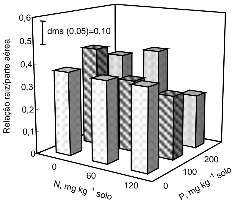
Figura 31. Efeito da adição de N e P no solo sobre a relação raiz/parte aérea de mudas de Sclerobium paniculatum em Latossolo Vermelho Escuro aos 230 dias após a semeadura (dms = diferença mínima significativa ao nível de 5%).
