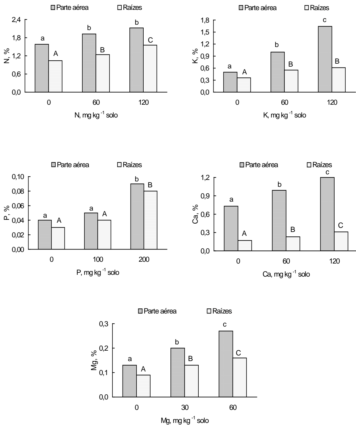
Figura 62. Efeito da adição de N, P, K, Ca e Mg no solo sobre a concentração do próprio elemento na parte aérea e nas raízes de mudas de Hancornia speciosa em Latossolo Vermelho Escuro aos 170 dias após a semeadura. Médias seguidas pela mesma letra para o mesmo componente não diferem significativamente pelo teste de Tukey a 5%.
