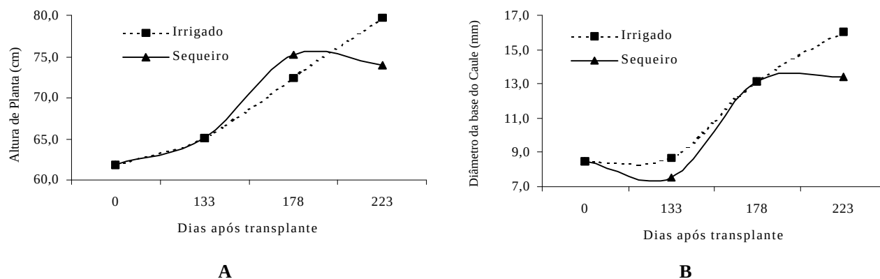
Figura 2 - Comportamento da altura de planta (A) e do diâmetro da base do caule (B) de Coffea arabica L. cv. Acaiá Cerrado MG 1474 em dois regimes hídricos e três épocas de avaliação, após transplante, no período de março a junho de 2001, (Brasília - DF).
