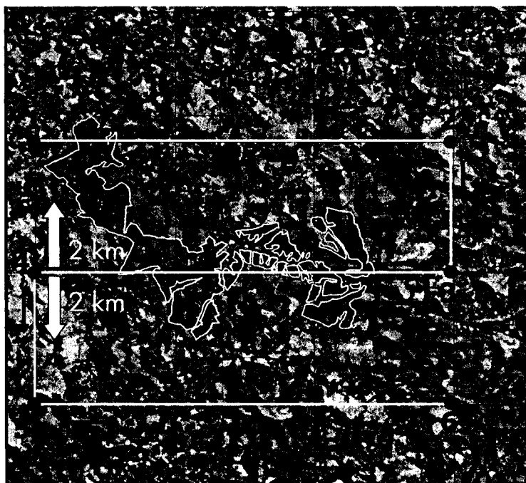
Figura 5 – Recorte de carta-imagen de una región sobrevolada con la técnica de LAE en el centro de la Provincia de Paraná, con las líneas de vuelo señaladas en blanco
