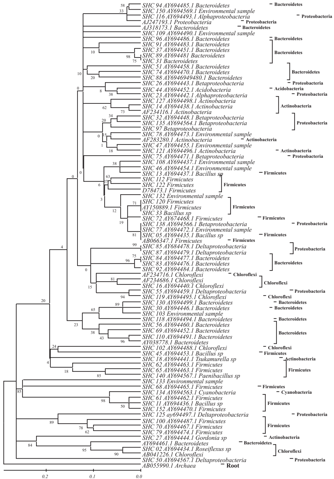
Figura 2 - Relacionamento filogenético baseado na amplificação da região 16S rDNA através de PCR de amostras do solo SHC, a árvore foi enraizada com a sequência de Archaea
