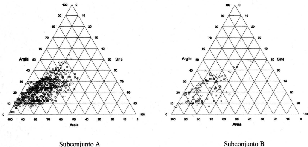
Figura 2. Classificação textural das amostras de solo utilizadas pra estimação (A) e validação (B) das PTFs
