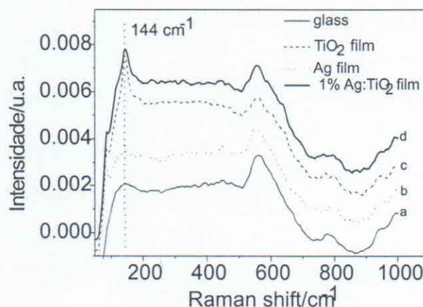
Fig. 1. Espectros Raman para os filmes com 4 camadas de Ag, \text{TiO}_2 e \text{TiO}_2 : 1% Ag
