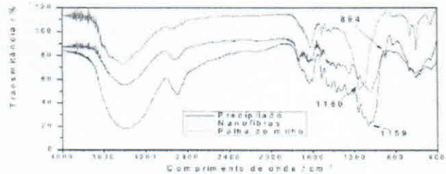
Fig. 4. FTIR da palha de milho, da nanocelulose obtida de palha de milho e do precipitado da reação de hidrólise.
