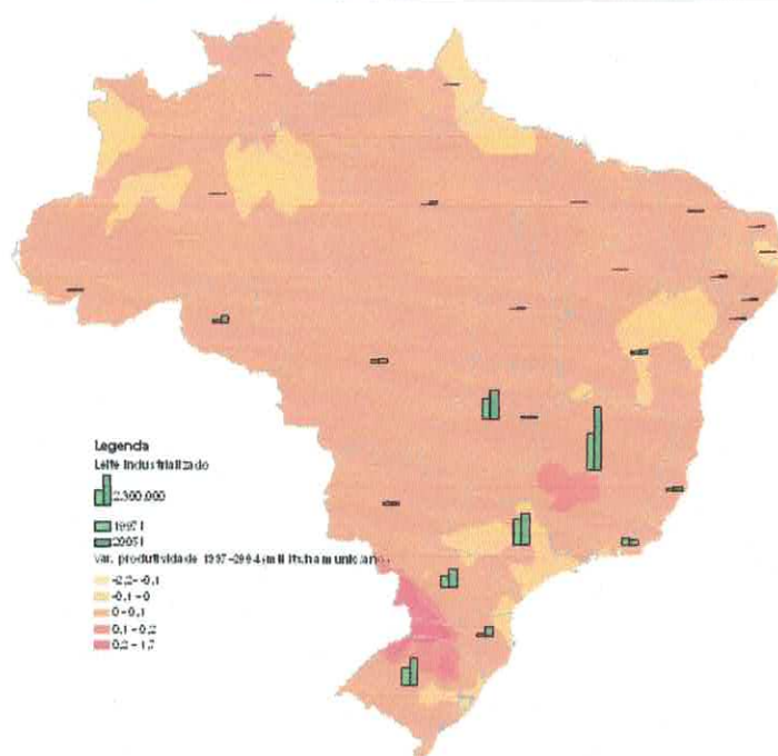
Figura 3 – Regiões de adensamento da produção primária de leite entre 1997 e 2004 e crescimento da industrialização de leite e derivados entre 1997 e 2005.
