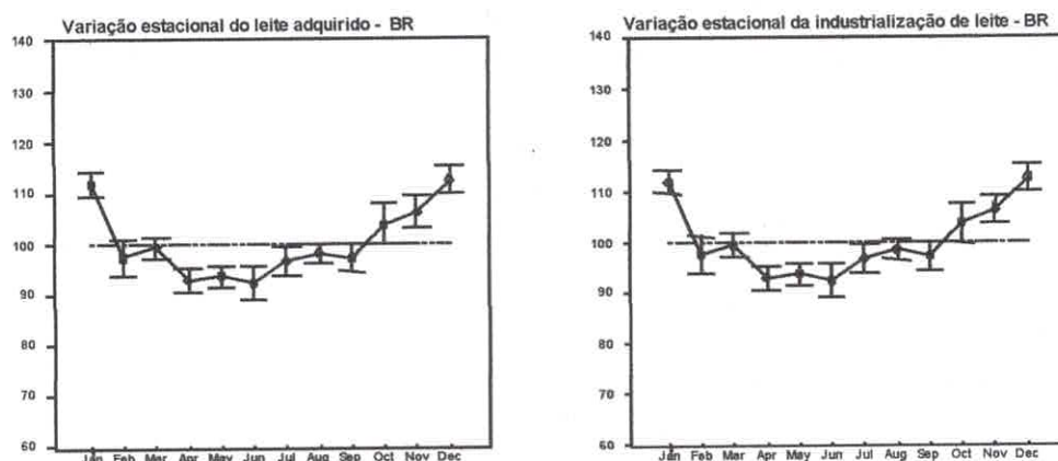
Figura 1 – Índices sazonais para os volumes de leite cru adquirido e industrializado no Brasil, para o período de 1997 a 2005.
