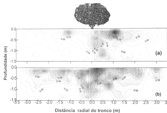
FIGURA 4 - Distribuição de densidade de comprimento de raízes (cm.cm -3 ) em dois perfis (a) na direção ortogonal a fileira de plantas, (b) na direção longitudinal a fileira de plantas, sob sistema de irrigação de microaspersão.
