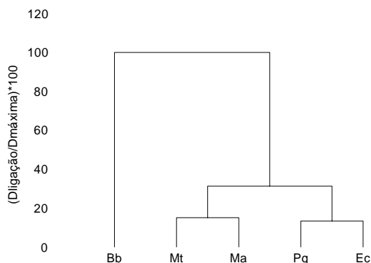
Figura 2. Dendrograma associado às similaridades dos teores de polifenóis, de N, e da relação C:N, como variáveis de caracterização do ambiente no solo sob a copa das leguminosas e do pasto solteiro (Bb- Brachiaria brizantha ; Mt- Mimosa tenuiflora ; Ma- Mimosa artemisiana ; Pg- Pseudosamanea guachapele ; Ec- Enterolobium contortisiliquum ).
