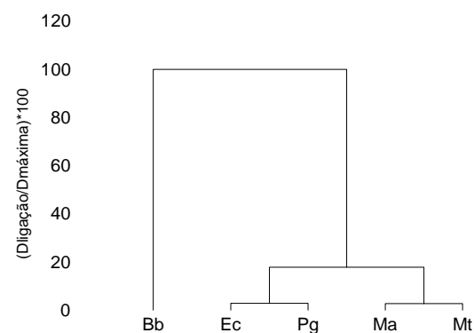
Figura 1. Dendrograma associado às similaridades das densidades dos grupos taxonômicos como variáveis de caracterização do ambiente no solo sob a copa das espécies leguminosas e do pasto solteiro (Bb- Brachiaria brizantha ; Mt- Mimosa tenuiflora ; Ma- Mimosa artemisiana ; Pg- Pseudosamanea guachapele ; Ec- Enterolobium contortisiliquum ).
