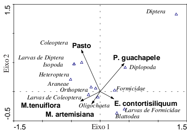
Figura 3. Diagrama de ordenamento obtido a partir da análise fatorial de correspondência, utilizando as densidades dos grupos taxonômicos da macrofauna como variáveis para caracterização do ambiente no solo sob as copas das leguminosas e no pasto solteiro (Eixo 1 = 37,3% da variância explicada; Eixo 2 = 26,1% da variância explicada).
