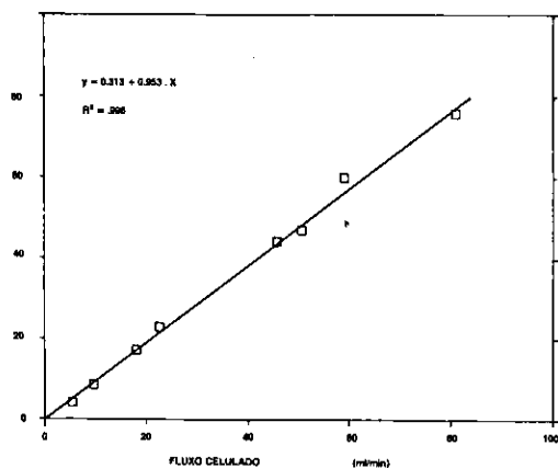
FIG. 5. Regressão linear relacionando fluxo de ar calculado com a equação 2 e fluxo medido com o bolhômetro. O fluxo de ar do capilar de referência foi 403 ml/min a 23 \pm 0.5^\circ\text{C} , sob um gradiente de pressão de 60 cm de coluna de água no baróstato.
