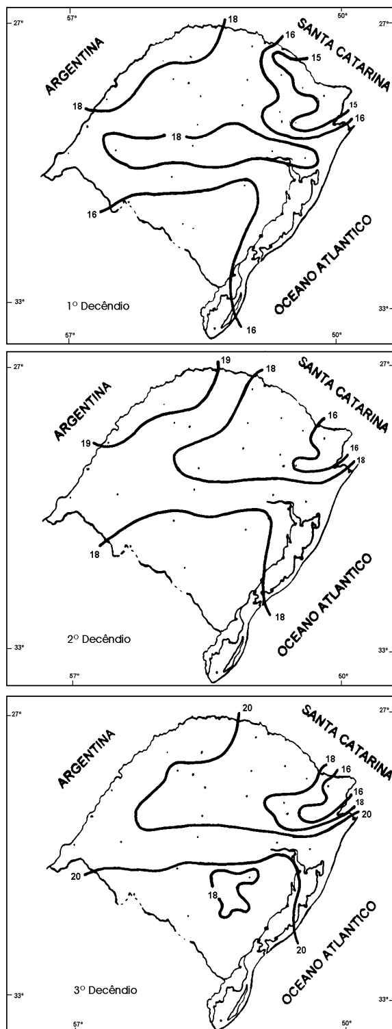
Figura 3. Temperatura ( ^{\circ}\text{C} ) do solo desnudo a 5 cm de profundidade do 1º, 2º e 3º decênio do mês de SETEMBRO , no estado do Rio Grande do Sul.
