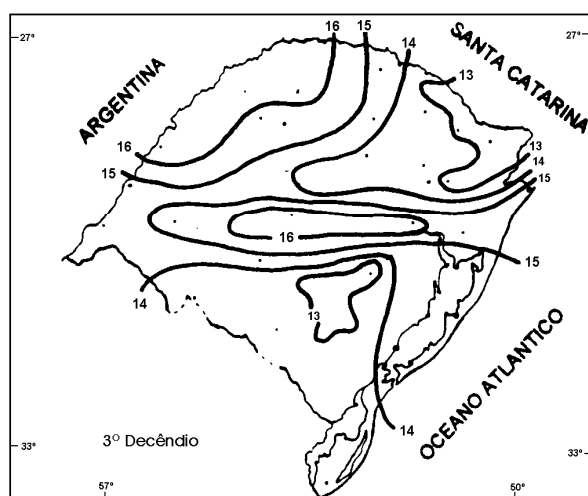
Figura 1. Temperatura (°C) do solo desnudo a 5 cm de profundidade do 1º, 2º e 3º decêndio do mês de JULHO , no estado do Rio Grande do Sul.
