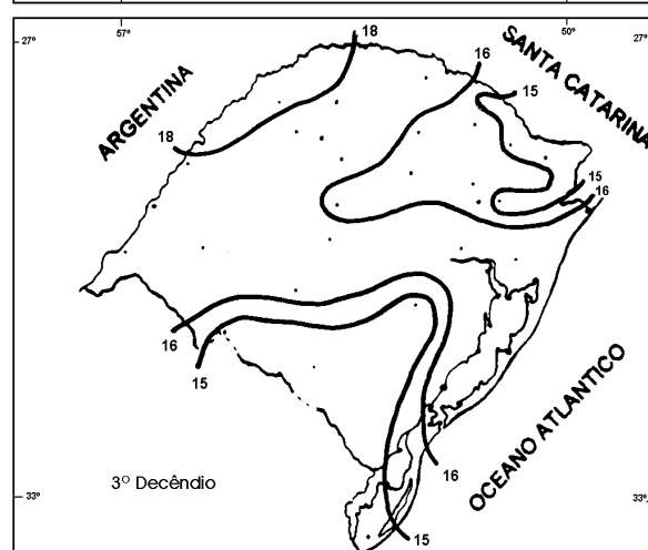
Figura 2. Temperatura (°C) do solo desnudo a 5 cm de profundidade do 1º, 2º e 3º decêndio do mês de AGOSTO , no estado do Rio Grande do Sul.
