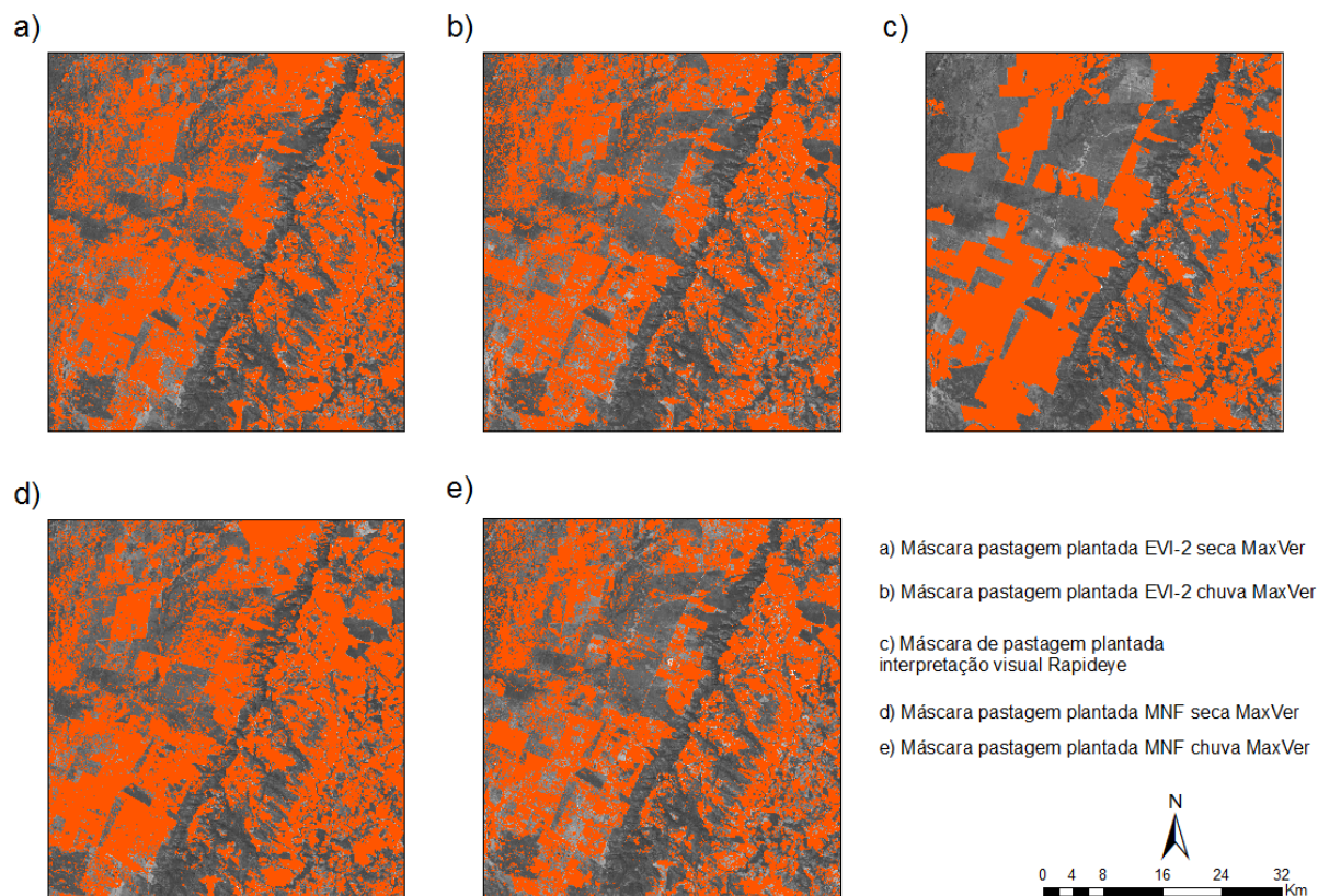
Figura 2. Resultado da classificação MAXVER da série temporal EVI-2 e EVI2-MNF e máscara de pastagem plantada obtida da imagem RapidEye, com banda 3 da imagem Landsat-5, de 20 de julho de 2011, ao fundo.
