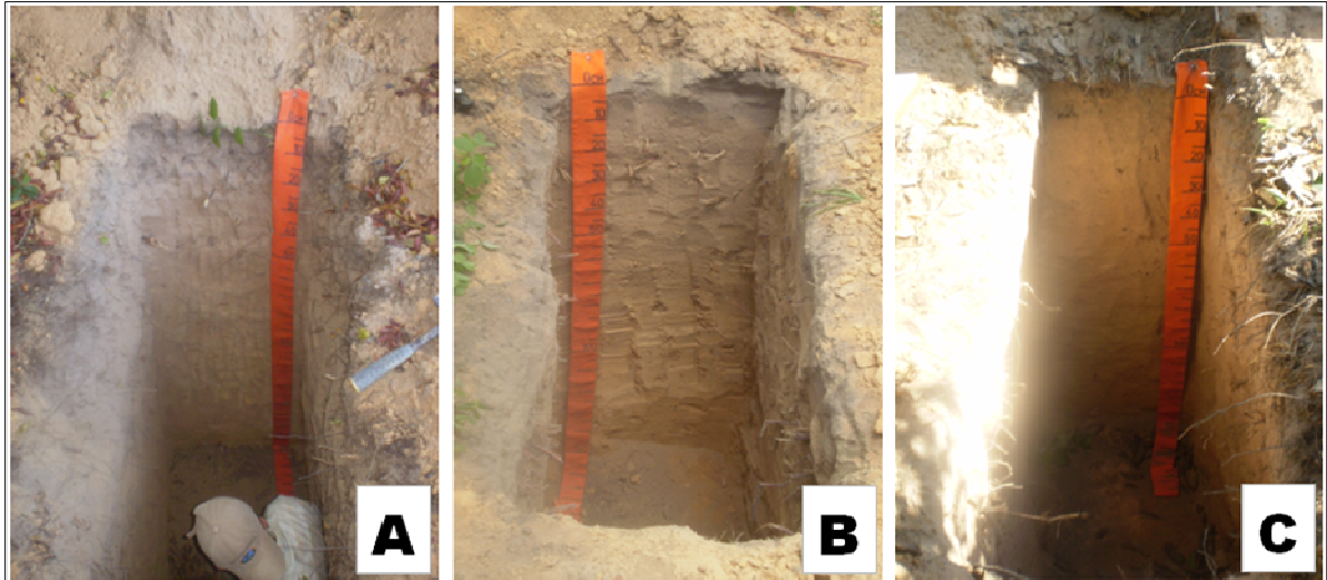
Figura 3. Trincheiras abertas nas áreas de estudo para caracterização do solo. A. Solo sob mata, B. Solo sob cultivo de coqueiros, C. Solo sob cultivo de graviroleiras.
