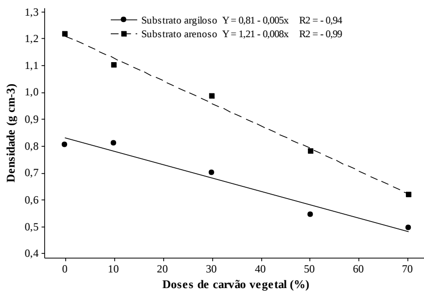
Figura 6 – Análise de regressão entre doses de carvão vegetal e a densidade do substrato, para substrato argiloso e arenoso.
