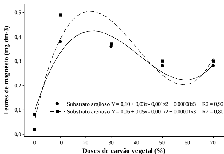
Figura 12 - Análise de regressão entre doses de carvão vegetal e teores de Mg para substratos argiloso e arenoso
