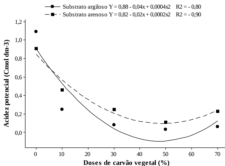
Figura 14 – Análise de regressão entre doses de carvão vegetal acidez potencial ( \text{H}+\text{Al} cmol dm -3 ), em substrato argiloso e arenoso.
