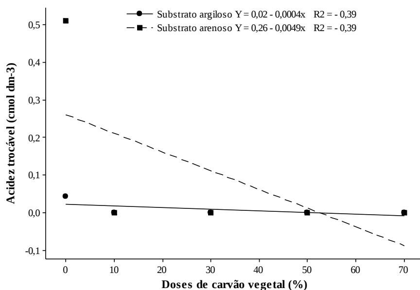
Figura 13 - Análise de regressão entre doses de carvão vegetal e \text{Al}^{3+} para substrato argiloso e arenoso
