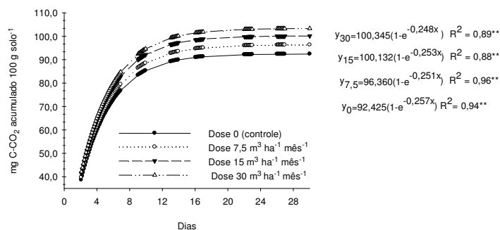
Figura 2. Quantidades de C-CO 2 acumulado liberado no período de 26 dias de incubação. Modelo ajustado para equação cinética de primeira ordem: y = a*(1 - e^{-kx}) , onde y_0 , y_{7,5} , y_{15} e y_{30} representam, respectivamente, o C-CO 2 estimado para os tratamentos controle sem adição e adição de 7,5 15 e 30 m 3 de efluente ha -1 mês -1 ; a = C potencialmente mineralizável; x = tempo de incubação e k = constante de velocidade de reação de mineralização de C, em dias -1 . (** Significativo a 1% de probabilidade)
