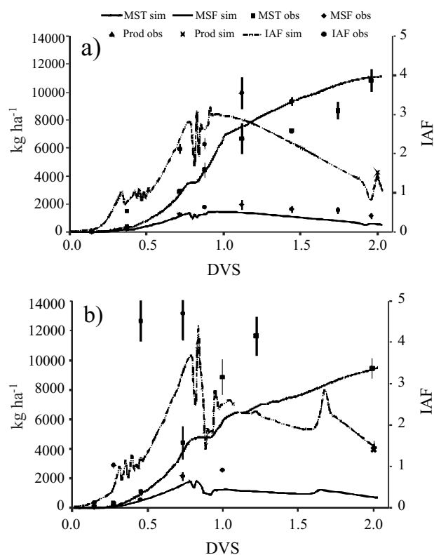
Figura 6 - Valores - observados (obs) e simulados (sim), pelo modelo ORYZA-APSIM, das variáveis (matéria seca total - MS_p , \text{kg ha}^{-1} ; matéria seca das folhas - MS_f , \text{kg ha}^{-1} ; índice de área foliar - IAF , \text{m}^2 \text{m}^{-2} ; produtividade - Prod , \text{kg ha}^{-1} ) para os experimentos a) 1 e b) 2 em função do tempo cronológico do modelo (DVS)
