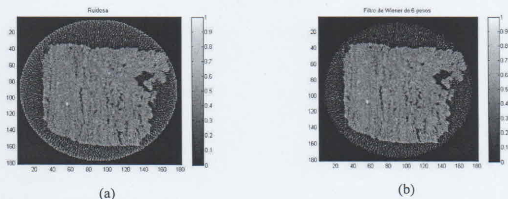
FIGURA 3. Análises de uma amostra de Latossolo Vermelho-Escuro reconstruídas com o uso da técnica de tomografia de raios-X para análise de densidade. (a) Imagem com ruído Poisson; (b) Imagem filtrada com filtro de Wiener por predição linear com 6 pesos.
