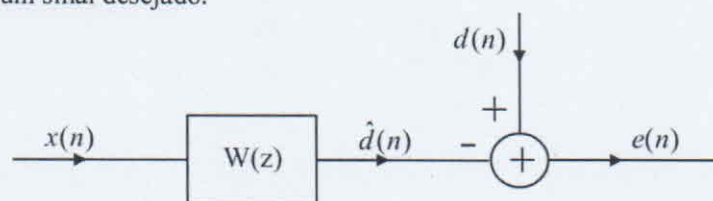
FIGURA 1. Ilustração de um problema geral do filtro de Wiener.
