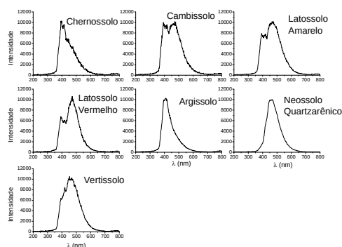
Figura 1 – a: Formação do excímero de pireno a partir de seus monômeros; b) espectros de emissão de fluorescência de pireno na concentração de 25 \mu\text{mol g}^{-1} em solo sem matéria orgânica.
