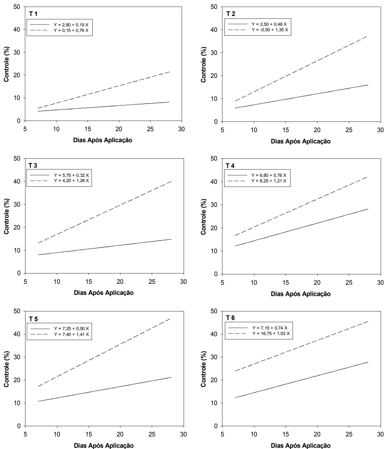
Figura 1. Eficiência de controle de plantas adultas de capim-mombaça em função de dias após aplicação de doses de glyphosate, sendo (—) 2,0 L ha -1 , e (- - -) 4,0 L ha -1 de glyphosate p.c., associadas a diferentes adjuvantes, sendo (T1) Sil01 0,5% v v -1 ; (T2) Sil01 50mL ha -1 ; (T3) Nit01 0,5% v v -1 ; (T4) assist 0,5% v v -1 ; (T5) sulfato de amônio 1,0% v v -1 ; (T6) ureia 0,5% v v -1 . Todos os valores de R 2 foram superiores a 0,9900. Doses do produto comercial por hectare. Formulação do glyphosate utilizada: sal de isopropilamina 480 g L -1 , equivalente ácido de N-(fosfometil) glicina 360 g L -1 . Embrapa Agropecuária Oeste, Dourados-MS, 2011.
