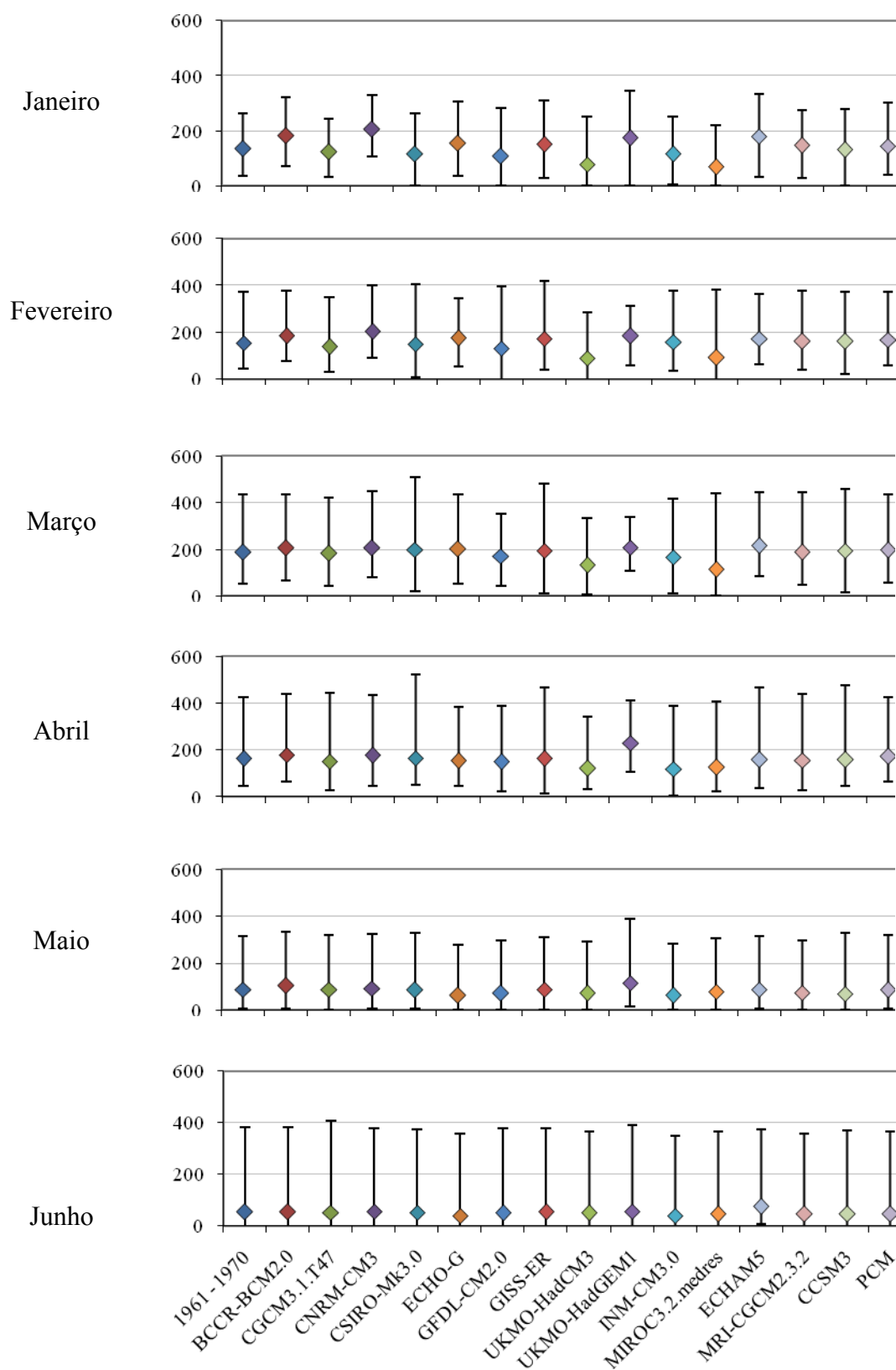
Figura 2. Precipitação média mensal (mm) de janeiro a junho da normal climatológica de 1961 a 1990 e de 15 modelos climáticos globais do período de 2071 a 2100, cenário A2 do IPCC-AR4 para a região Nordeste do Brasil. A barra vertical une os valores máximo e mínimo na região em cada mês e modelo.
