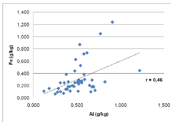
Figura 3. Correlação entre Al_o e Fei_o em todos os horizontes dos solos analisados.
