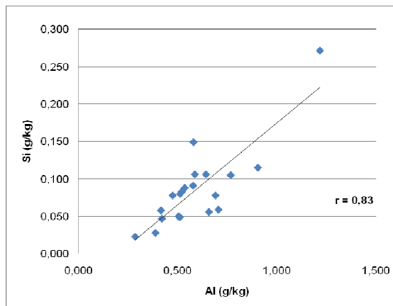
Figura 2. Correlação entre Al_o e Si_o nos horizontes coesos analisados.
