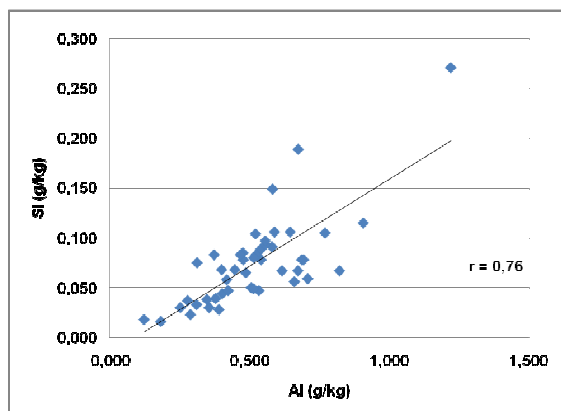
Figura 1. Correlação entre Al_o e Si_o em todos os horizontes dos solos analisados.
