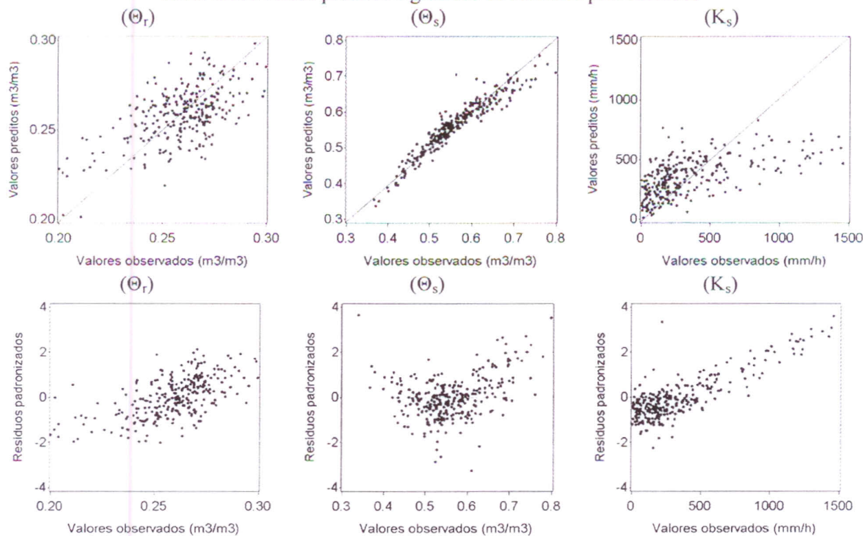
Figura 3- Padrões gráficos de resíduos das funções de pedotransferência ajustadas para as variáveis umidade residual, umidade de saturação e condutividade saturada, respectivamente: valores observados versus preditos e gráficos de resíduos padronizados
