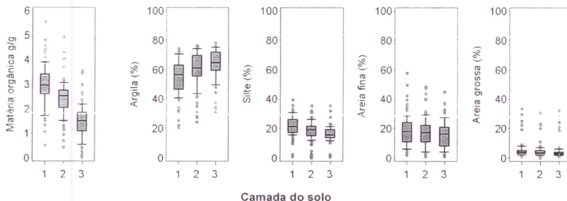
Figura 1- Variabilidade do conteúdo de matéria orgânica e propriedades texturais do solo, em três camadas de solo (1- 0-5cm; 2- 15-20cm; 3- 60-65cm), na área da bacia hidrográfica do rio Buriti Vermelho, DF.
