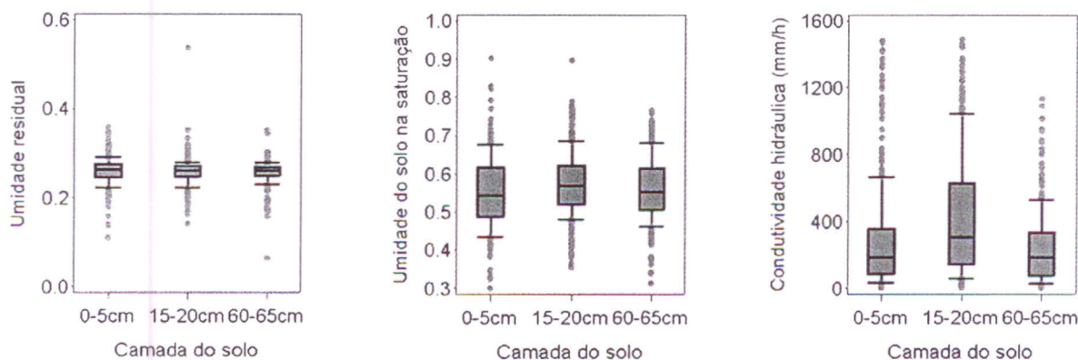
Figura 2- Variabilidade de propriedades hidráulicas do solo, em três camadas de solo, na área da Bacia Hidrográfica do Rio Buriti Vermelho, DF.
