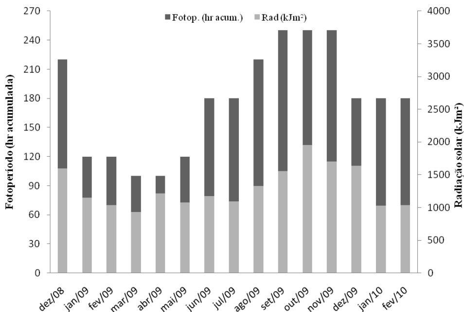
Figura 5. Médias mensais de fotoperíodo (Fotop., hr.) em horas e da radiação (Rad., kJ/m 2 ), ocorridas durante o período de dezembro de 2008 a fevereiro de 2010.
