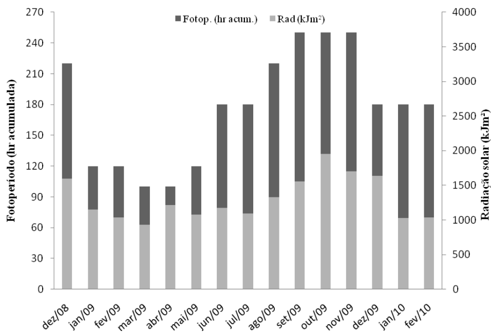
Figura 4. Médias mensais de fotoperíodo (Fotop., hr acum.) em horas e da radiação (Rad., kJ/m 2 ), ocorridas durante o período de dezembro de 2008 a fevereiro de 2010.
