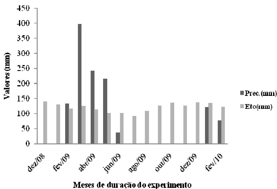
Figura 3. Médias mensais da precipitação (Prec) e Evapotranspiração potencial (Eto) ocorridas durante o período de dezembro de 2008 a fevereiro de 2010.
