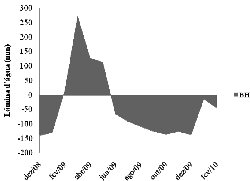
Figura 3. Médias mensais do Balanço Hídrico Climático (BH) ocorridas durante o período de Dezembro de 2008 a Fevereiro de 2010.
