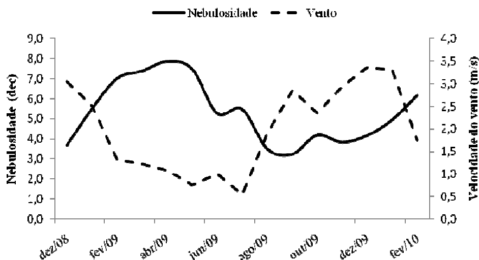
Figura 5. Médias mensais de Nebulosidade (dec; varia de 1 a 10 onde 1 é céu pleno sem nuvens e 10 céu completamente nublado) e velocidade do vento (m/seg), ocorridas durante o período de dezembro de 2008 a fevereiro de 2010.
