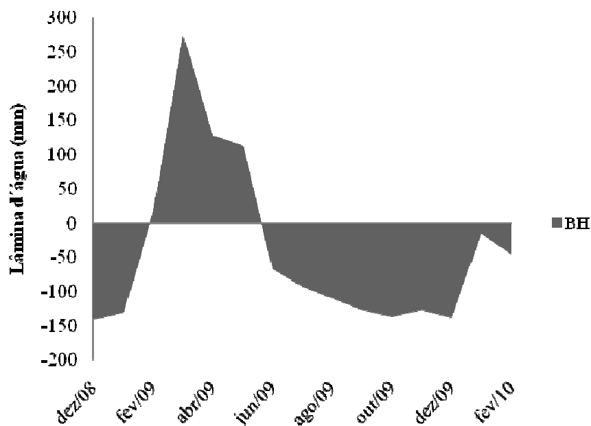
Figura 4. Médias mensais do balanço hídrico climático (BH) ocorridas durante o período de dezembro de 2008 a fevereiro de 2010.
