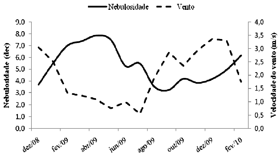
Figura 6. Médias mensais de nebulosidade (dec; varia de 1 a 10 onde 1 é céu pleno sem nuvens e 10 céu completamente nublado) e velocidade do vento (m/s), ocorridas durante o período de dezembro de 2008 a fevereiro de 2010.
