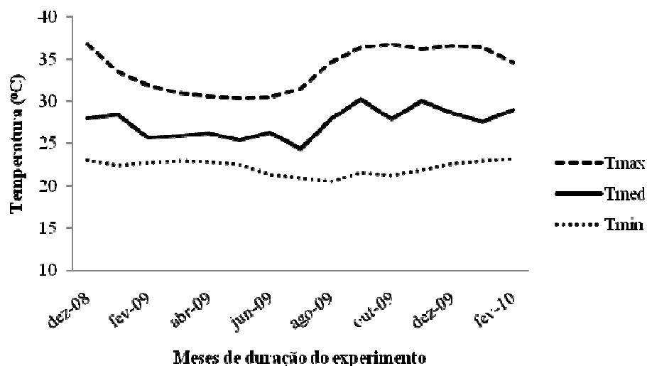
Figura 2. Médias mensais das temperaturas máxima (Tmax), média (Tmed) e mínima (Tmin) ocorridas durante o período de dezembro de 2008 a fevereiro de 2010.
