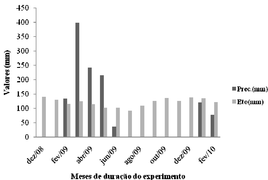
Figura 2. Médias mensais da Precipitação (Prec) e Evapotranspiração potencial (Eto) ocorridas durante o período de Dezembro de 2008 a Fevereiro de 2010.
