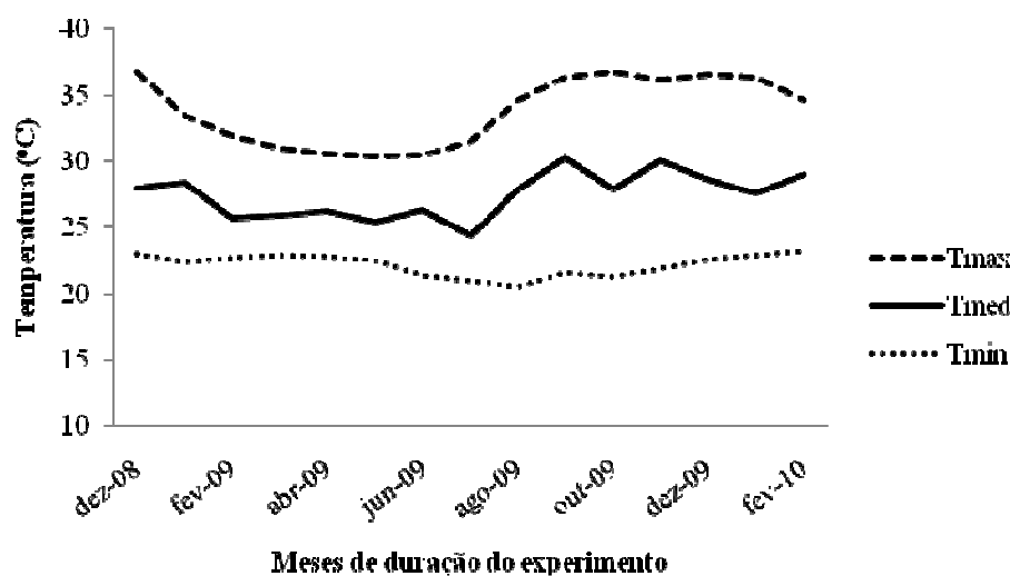
Figura 1. Médias mensais das temperaturas máxima (Tmax), média (Tmed) e mínima (Tmin) ocorridas durante o período de Dezembro de 2008 a Fevereiro de 2010.
