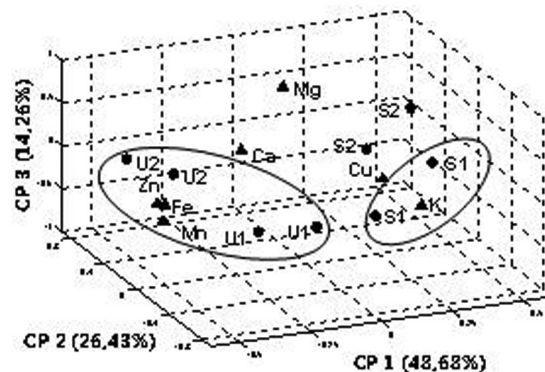
Figura 1. Gráfico bivariado ( biplot ) tridimensional de CP1 x CP2 x CP3. Os escores estão representados por círculos e os pesos por triângulos. S = digestão por via seca; U = digestão por via úmida; 1 = massa da amostra de 200 mg; 2 = massa da amostra de 500 mg
